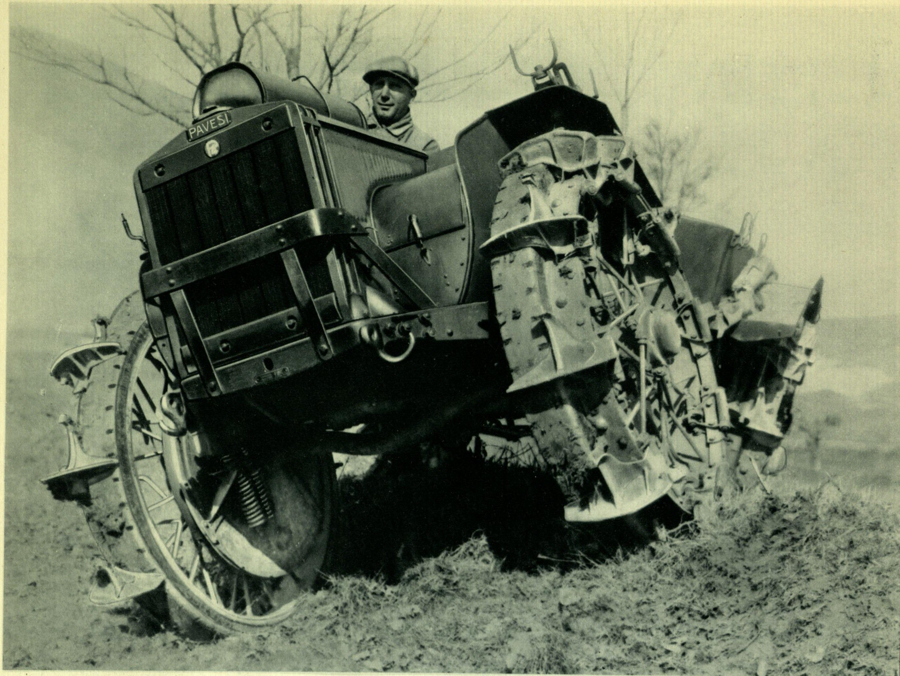
Trattore «Pavesi P 4».
