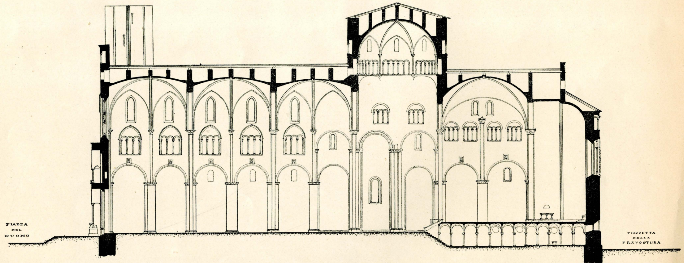
SEZIONE O PROFILO LONGITUDINALE DEL TEMPIO nel Secolo XIV.
