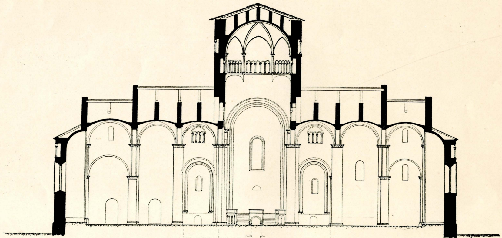
SEZIONE LONGITUDINALE DELLA TRASVERSA nel Secolo XIV.
