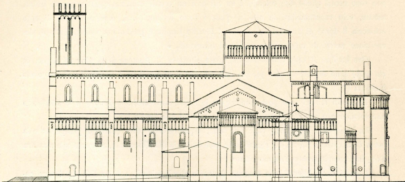
LATO O FIANCO A MEZZOGIORNO
