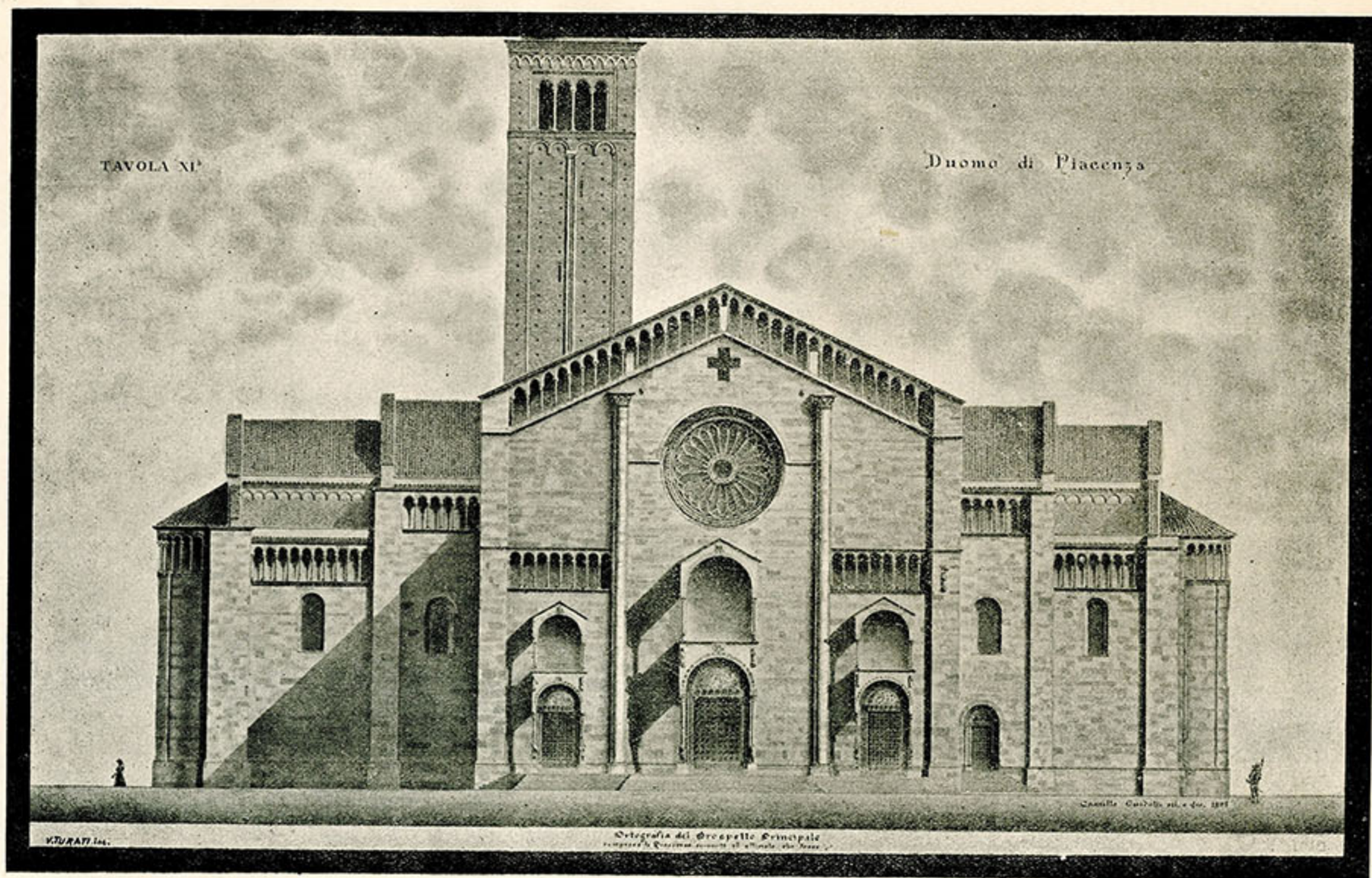
ORTOGRAFIA DEL PROSPETTO PRINCIPALE DEL TEMPIO compresa la Trasversa, scoperta ed ultimata che fosse, nel secolo XIV.
