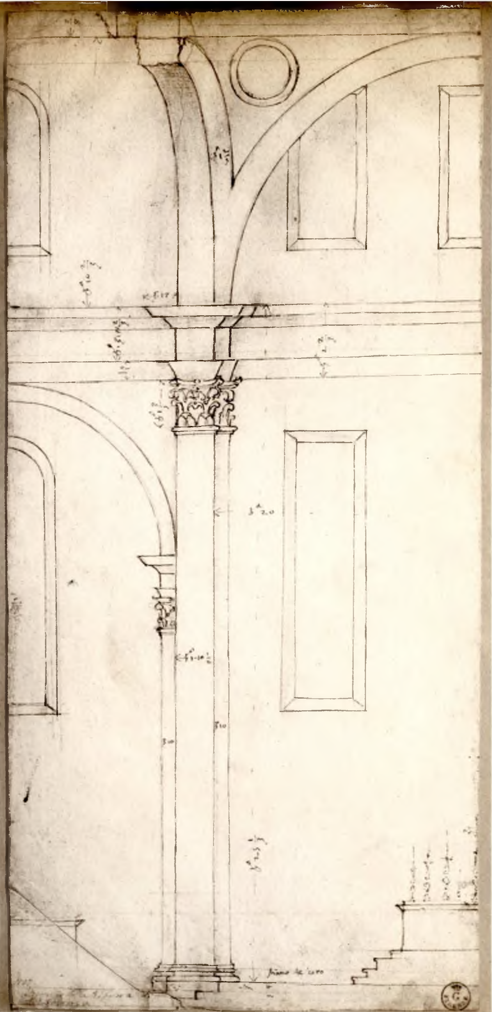
(Ed. ni Brogi 1000) UFFIZI - Disegni di Architettura. Tav. I - Brunelleschi (sec. XV)
