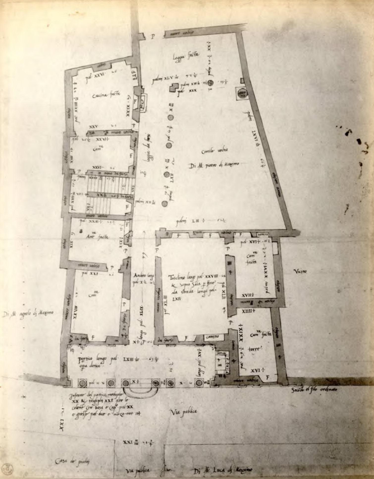
(Ed. n. Brogi 1042) UFFIZI - Disegni di Architettura, Tav. XLIII - Baldassarre Peruzzi (sec. XVI).
