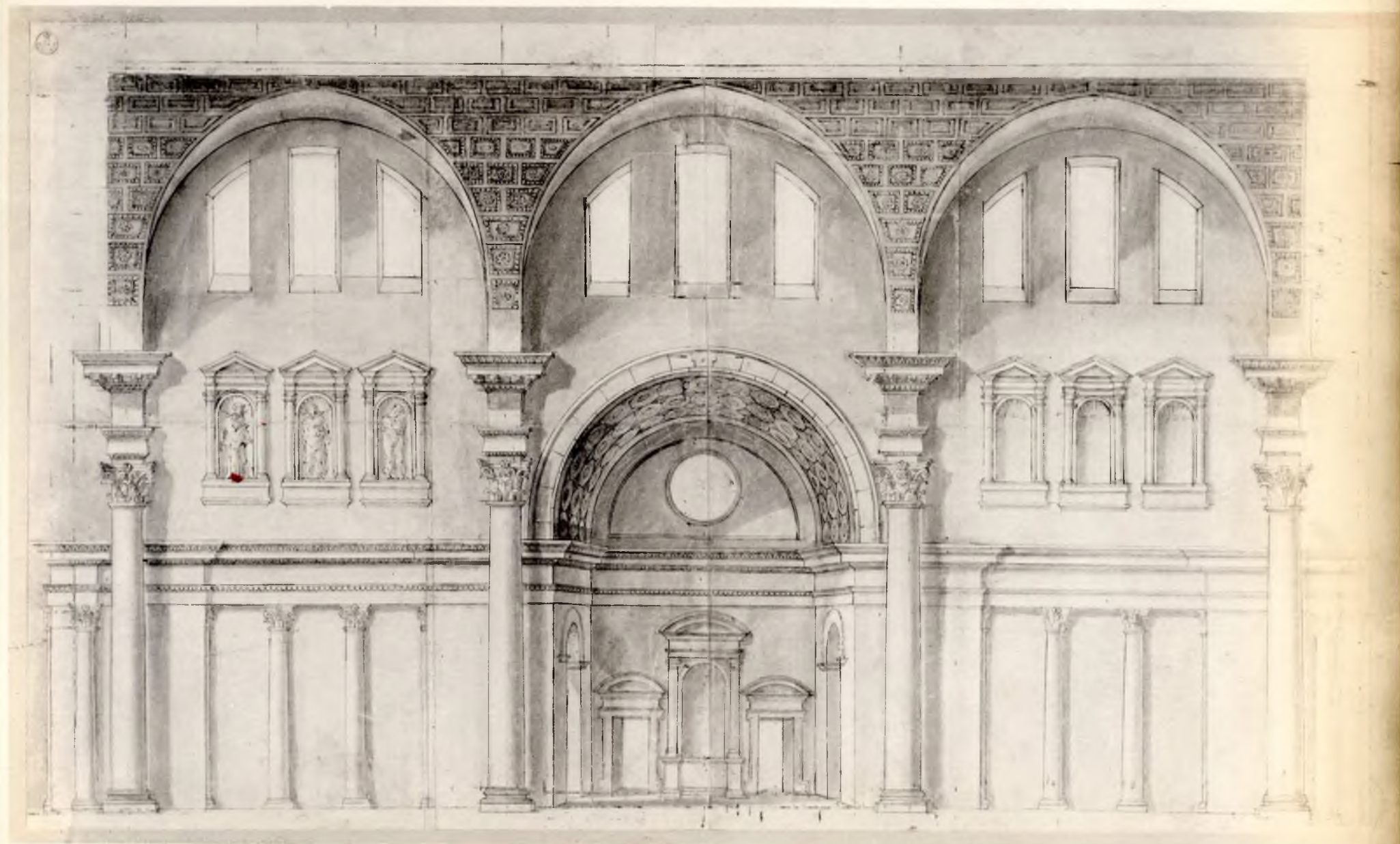
(Ed.ª Brogi 1016) UFFIZI - Disegni di Architettura, Tav. XVII - Giuliano da Sangallo (sec. XVI).
