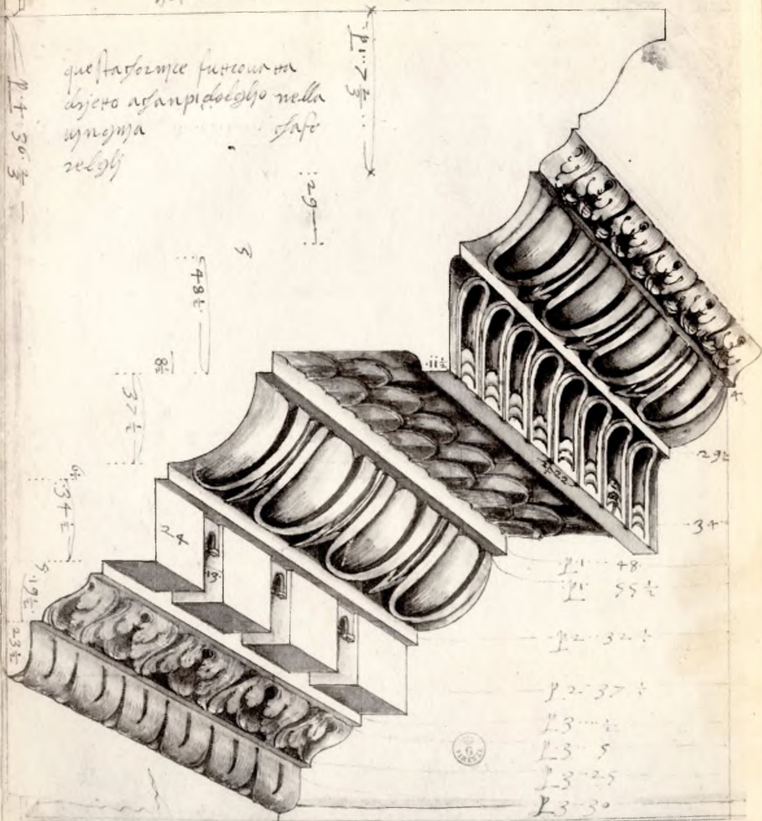
(Ed. n. Brogi 1028) UFFIZI - Disegni di Architettura, Tav. XXIX - Antonio da Sangallo (sec. XVI).
