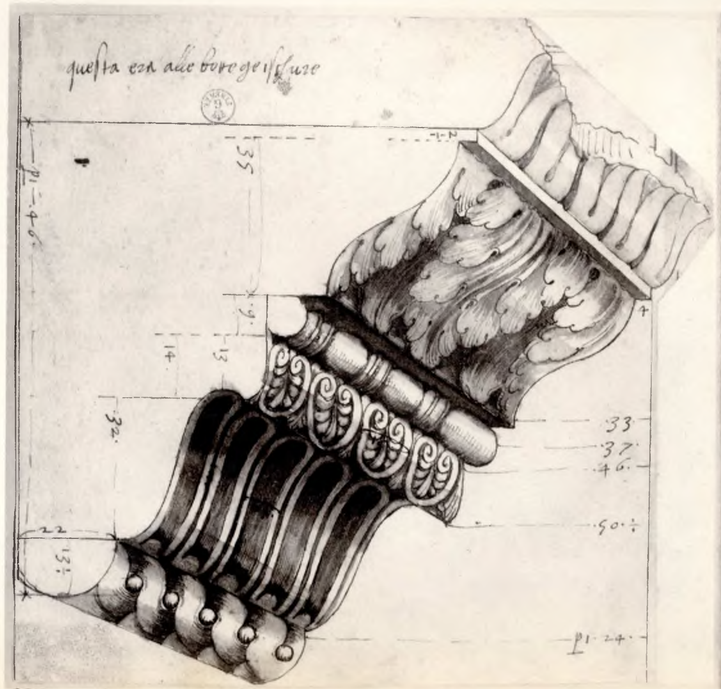
(Ed.ª Brogi 1029) UFFIZI - Disegni di Architettura, Tav. XXX - Antonio da Sangallo (sec. XVI).
