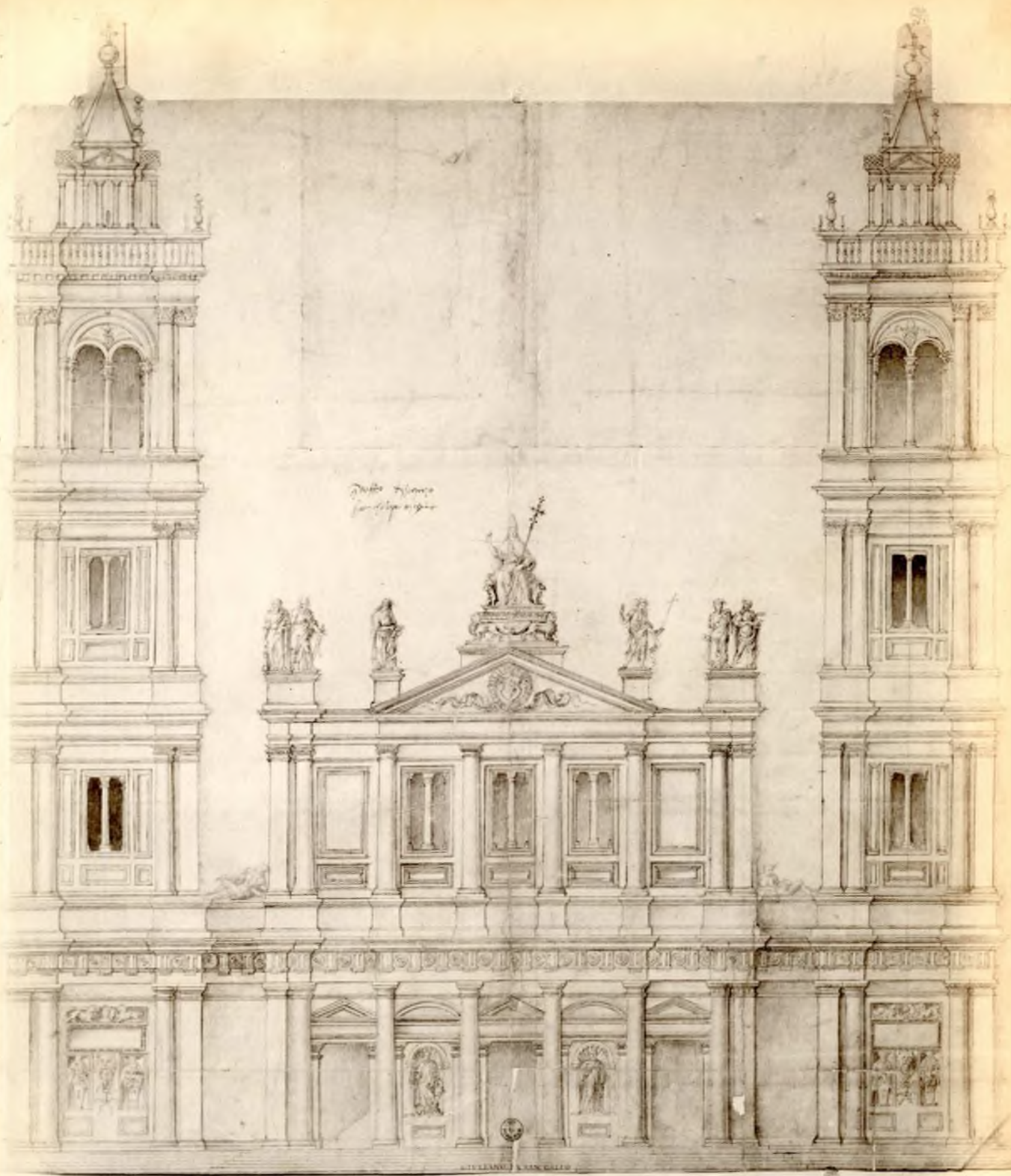
Facciata per la Chiesa di S. Lorenzo di Firenze
