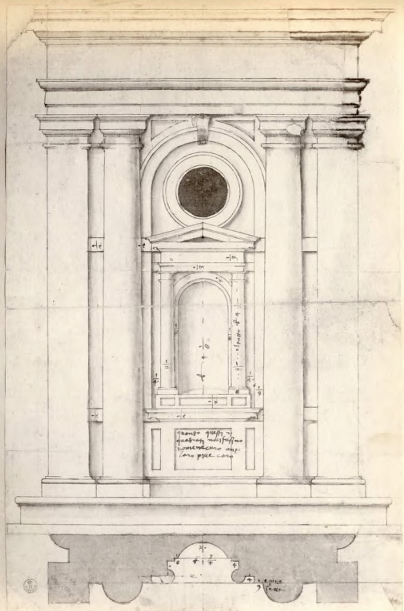
(Ed. n° Brogi 1027) UFFIZI - Disegni di Architettura. Tav. XXVIII - Antonio da Sangallo (sec. XVI).
