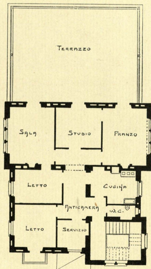
Primo piano.
