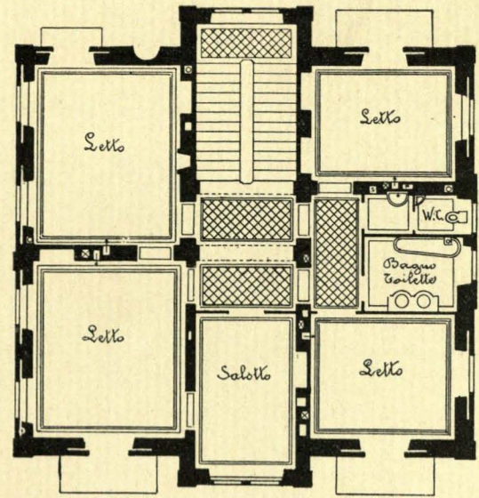
Primo piano.
