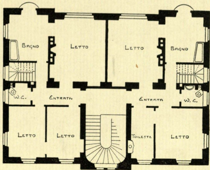
Primo piano.
