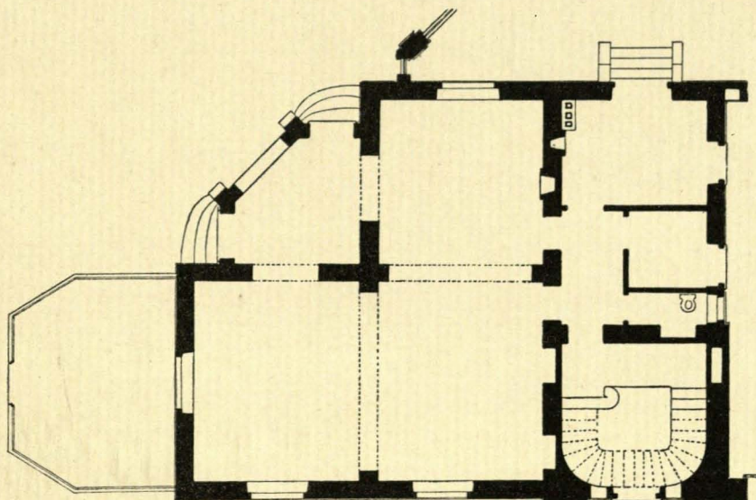
Piano terreno.
