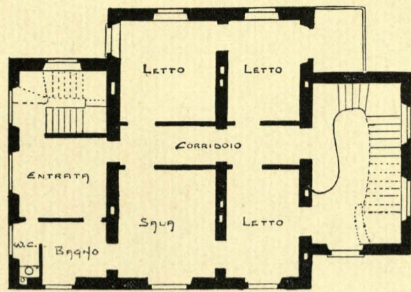
Primo Piano.
