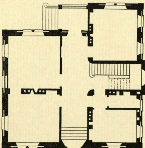
Piano terreno.
