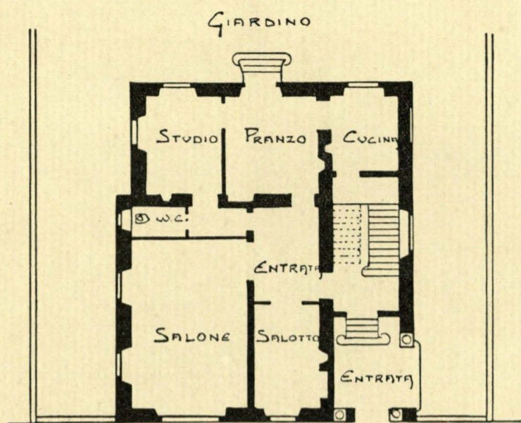
Piano terreno.
