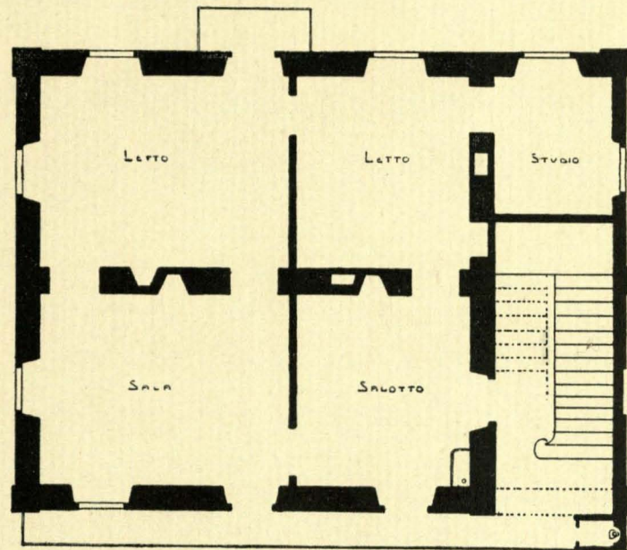
Primo piano.
