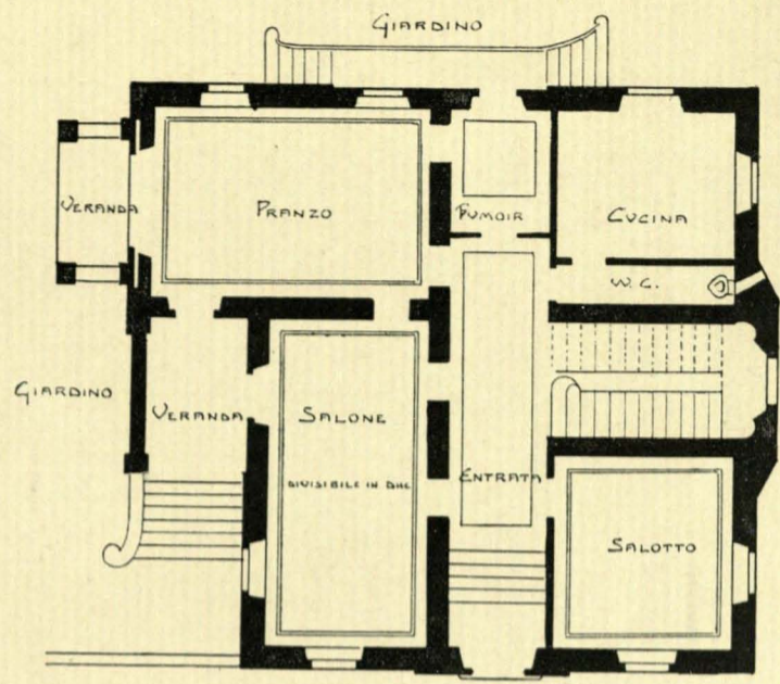
Piano terreno.
