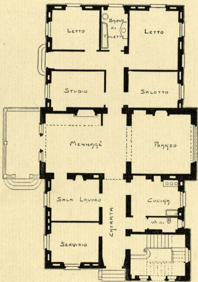
Piano terreno.
