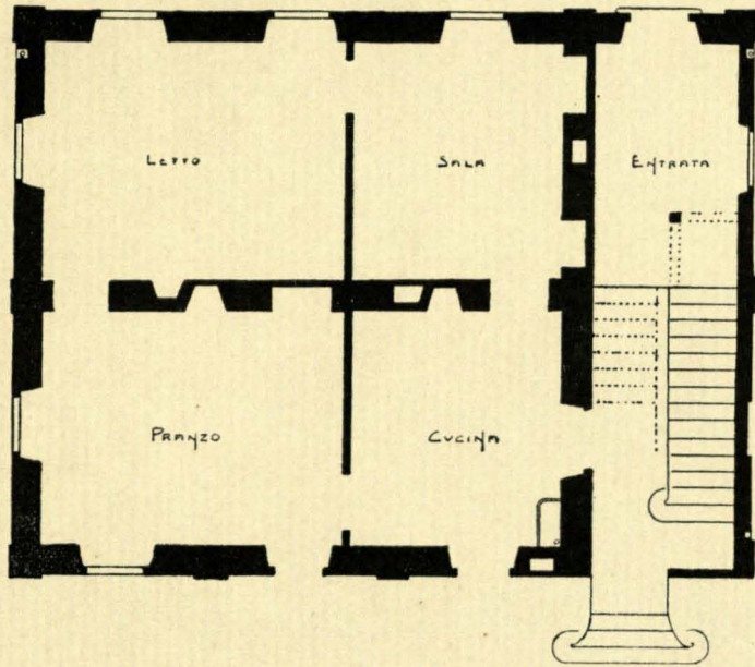
Piano terreno.
