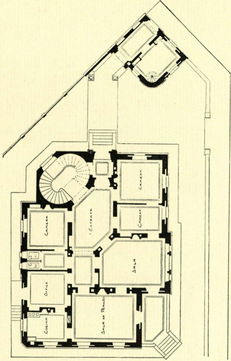
Primo e secondo piano.
