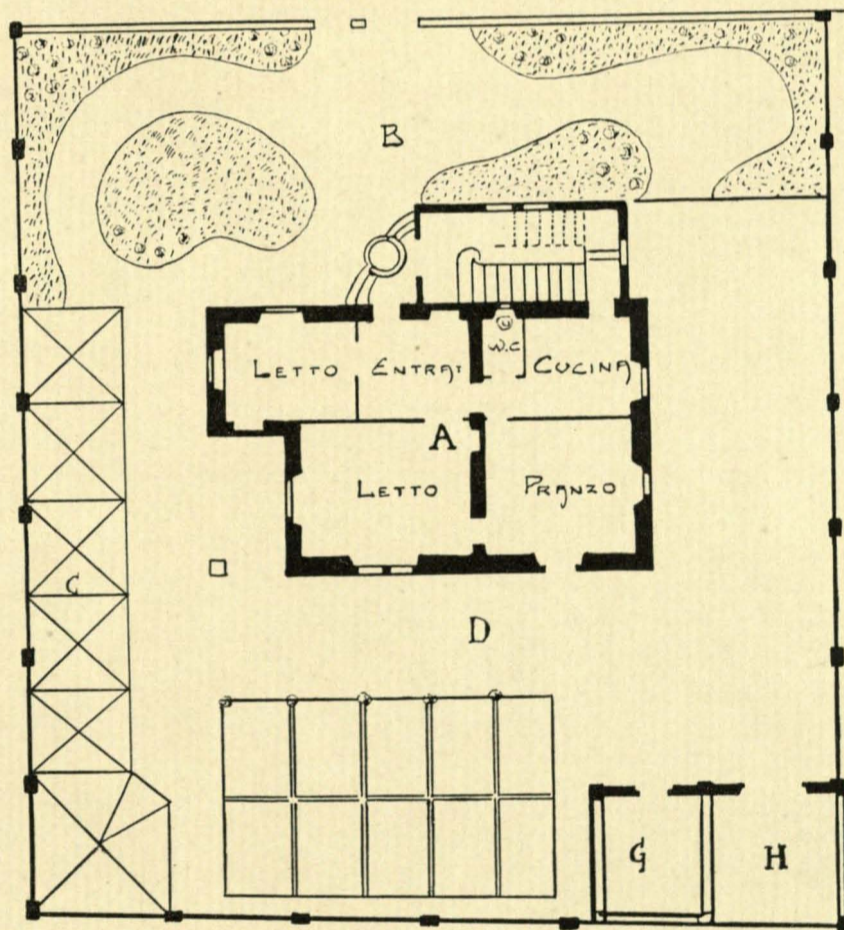
Piano terreno.
