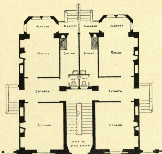
Piano terreno.
