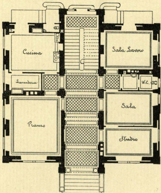
Piano terreno.
