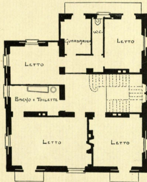
Primo piano.
