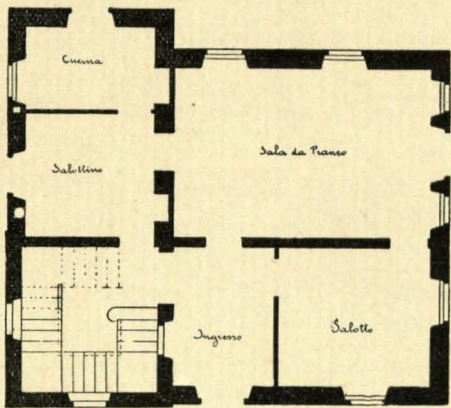
Piano terreno.
