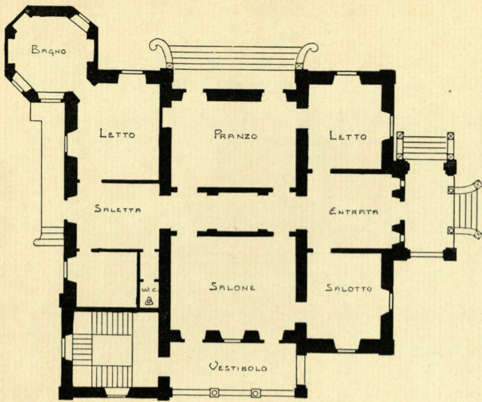
Piano terreno verso giardino e primo piano verso via.
