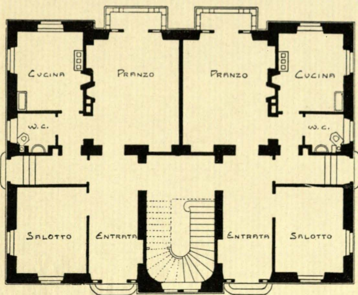
Piano terreno.
