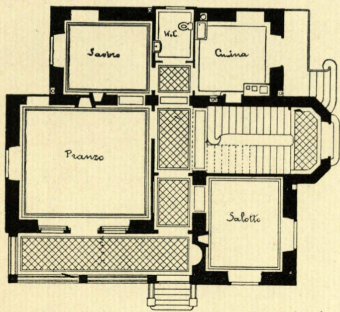
Piano terreno.
