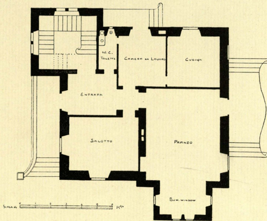
Piano terreno.
