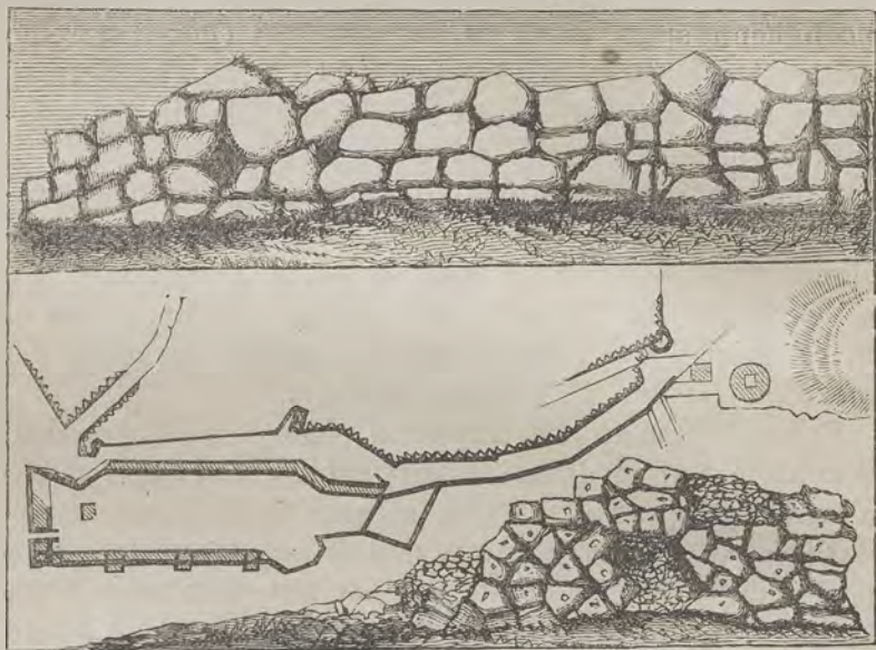
[Fortificazioni di Alba presso il lago Fucino ( Promis. ).
