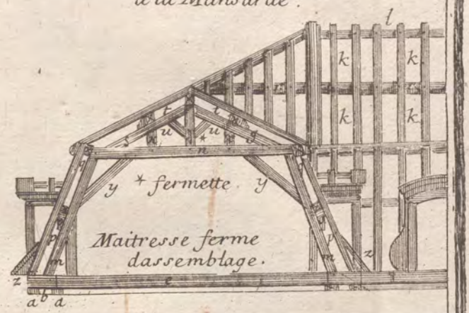
Profil et Courant du Comble a la Manarde.
