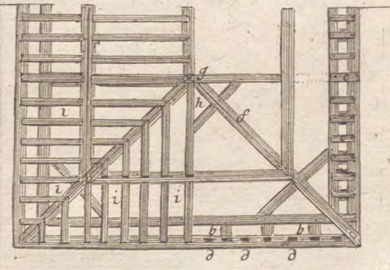
Plan de l'Enrayure
