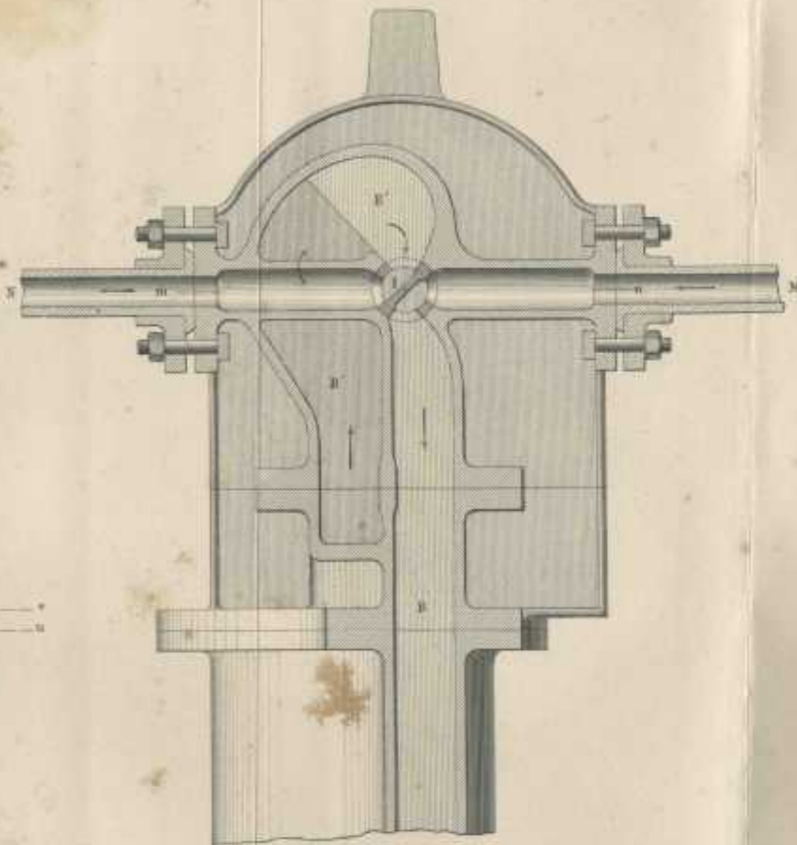
Fig. 4. Sezione orizzontale mn
