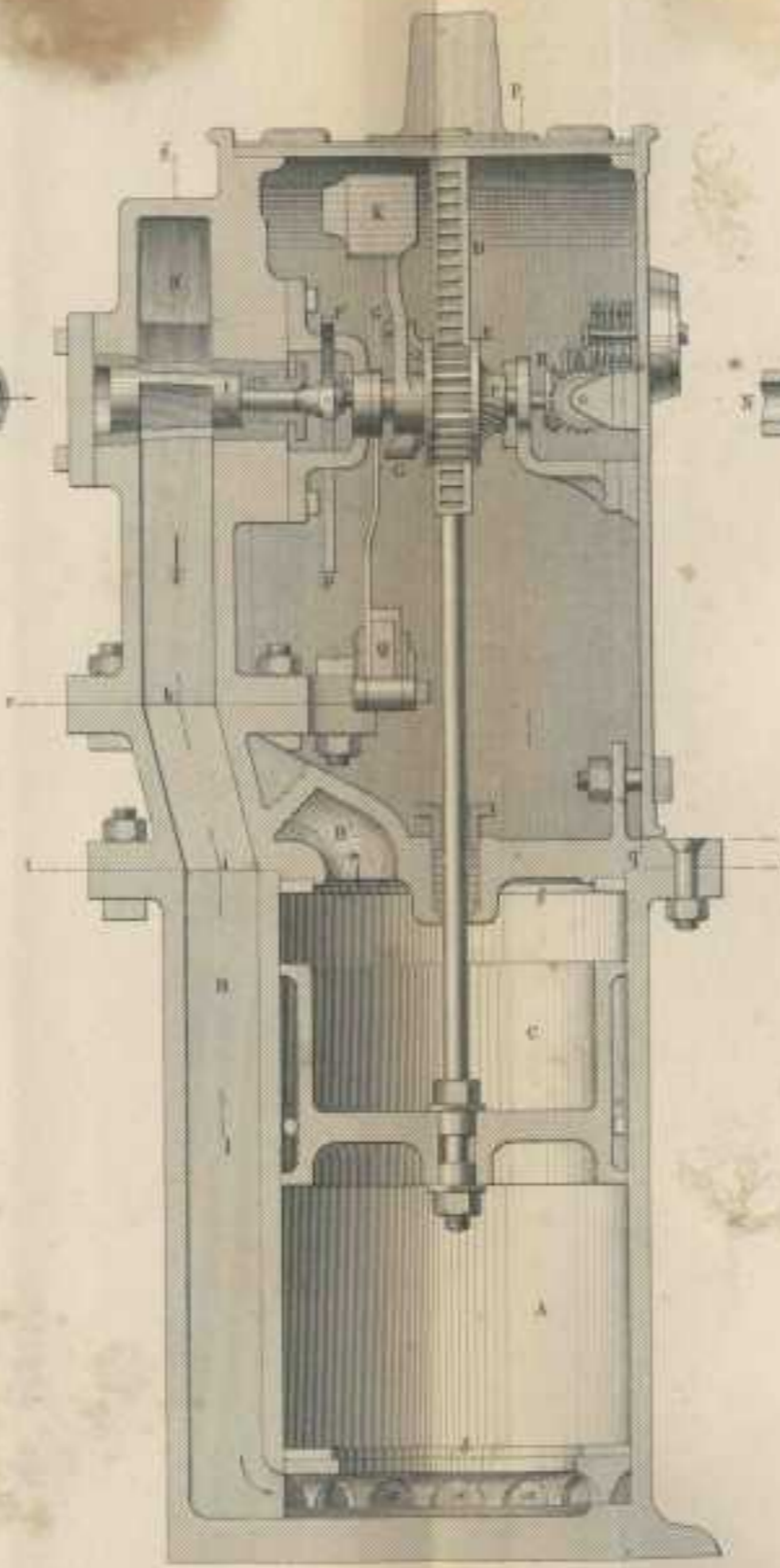
Fig. 2. Sezione verticale sull'asse del cilindro
