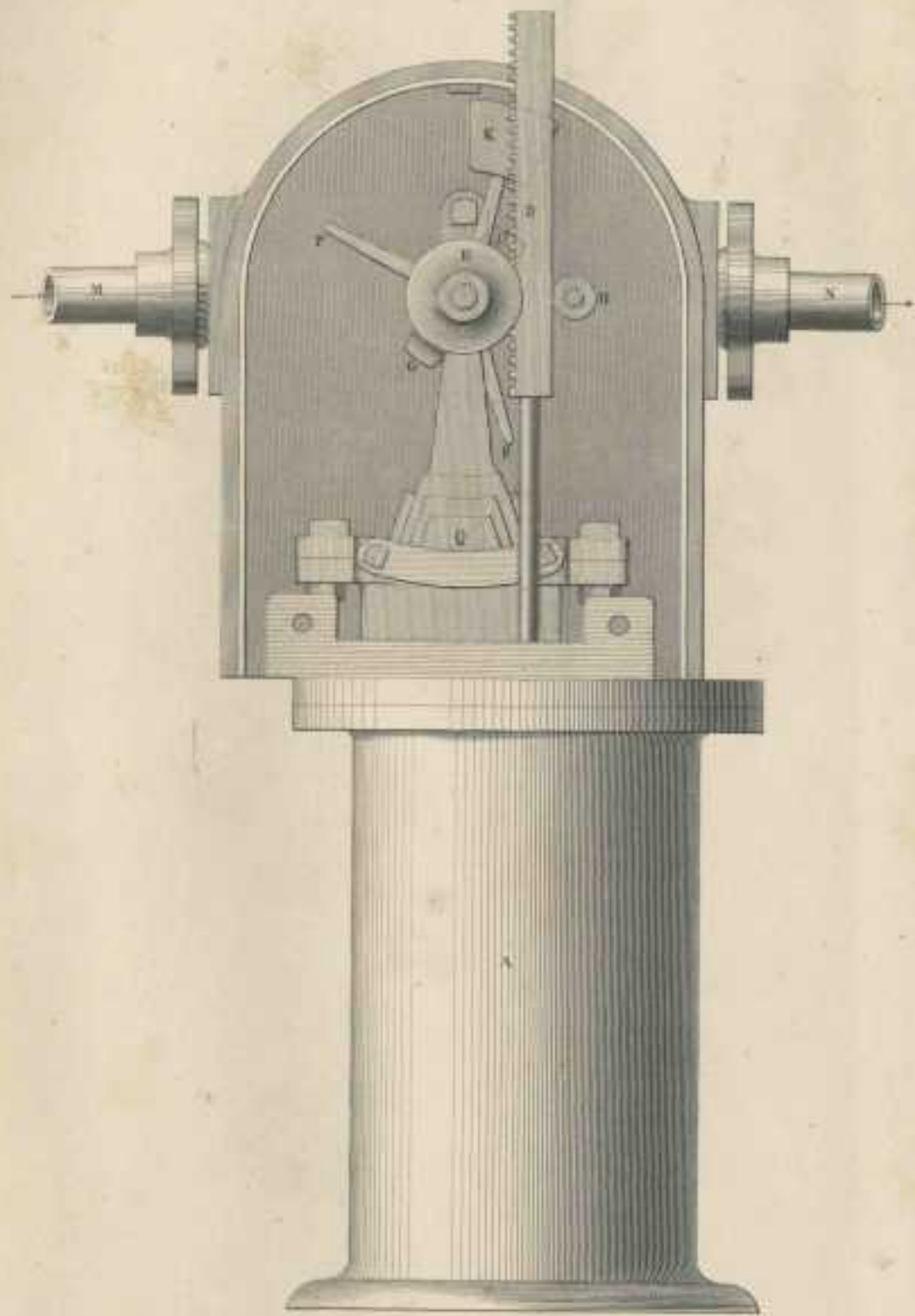
Fig. 5. Sezione verticale pq.
