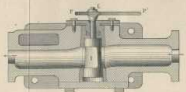
Fig. 4. Sezione orizzontale mn
