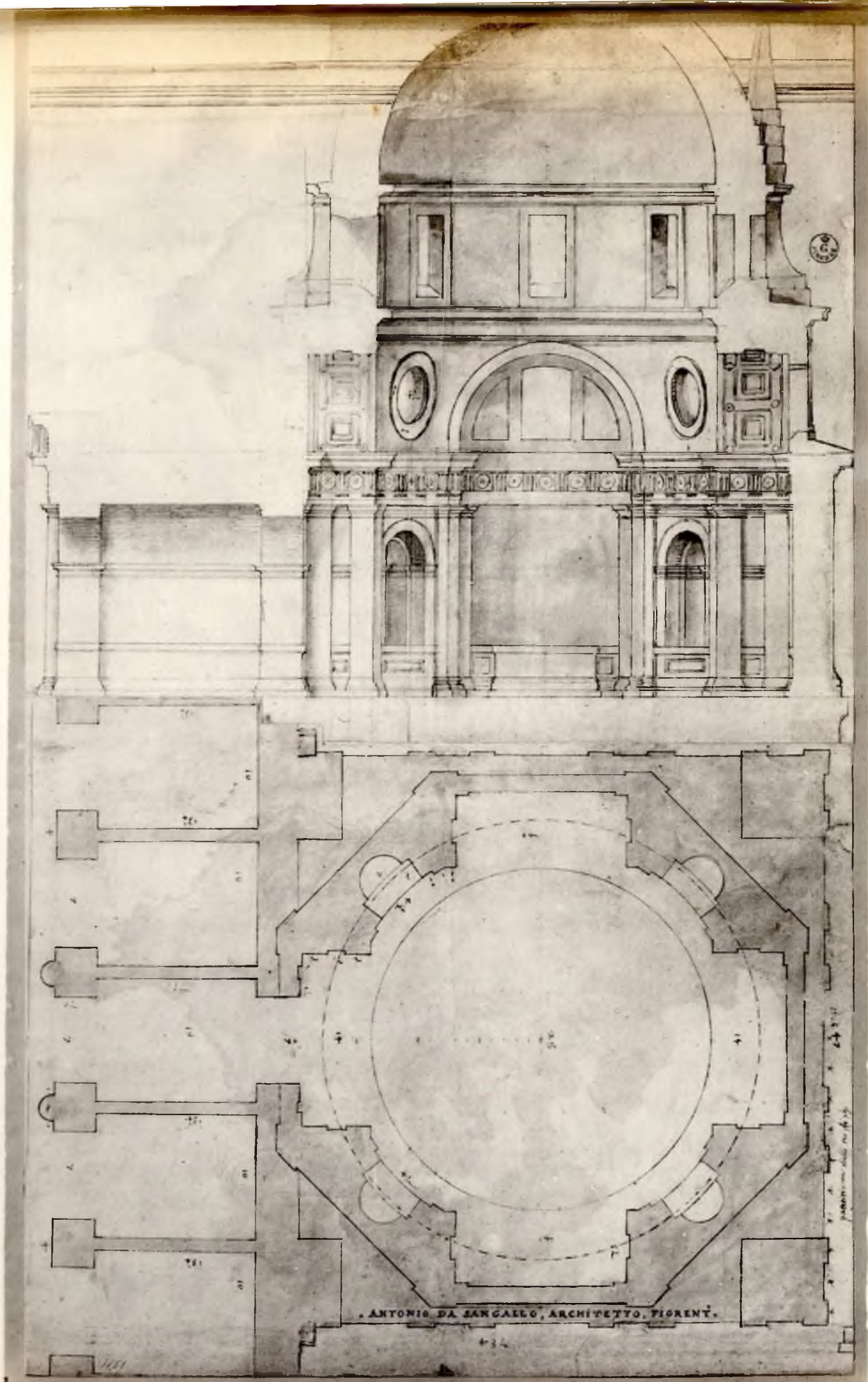
(Ed. ni Brogi 1060) UFFIZI - Disegni di Architettura, Tav. LXI - Antonio da Sannallo, il niiovine (sec. XVI).
