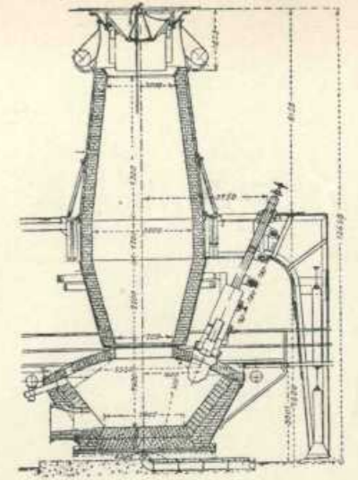
FIG. 15 - Alto Forno Svedese di 3000 KW di Hagfors.
