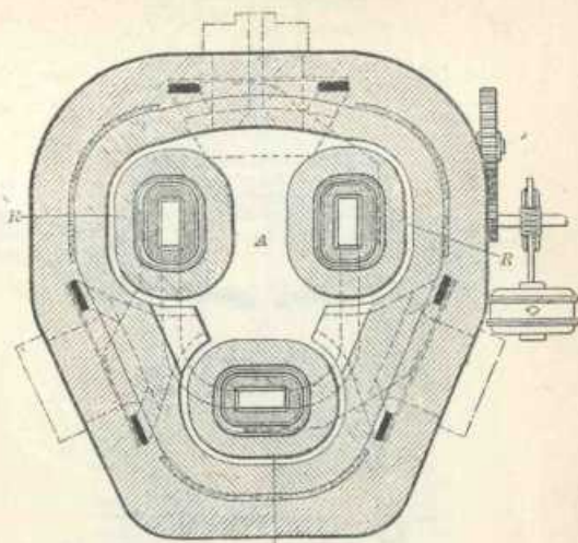
FIG. 4 - Forno trifase ad induzione Roechling (pianta).
