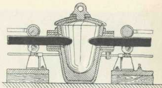
FIG. 5 - Fornetto Siemens ad arco indiretto.
