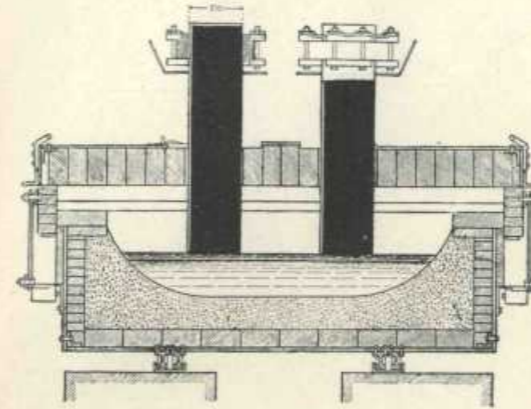
FIG. 13 - Forno ad arco diretto Héroult.
