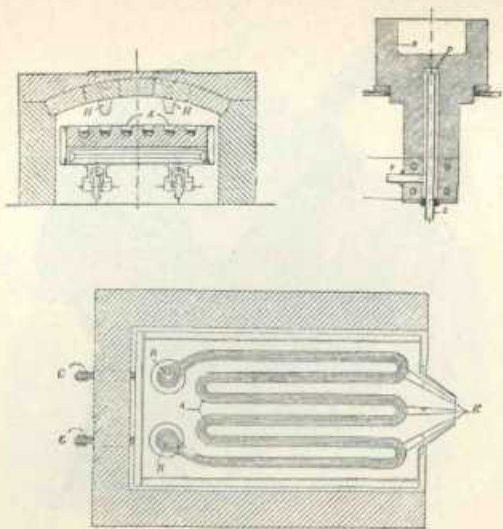
FIG. 1 - Forno a resistenza Gin.
