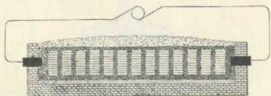
FIG. 2 - Forno a resistenza Acheson.
