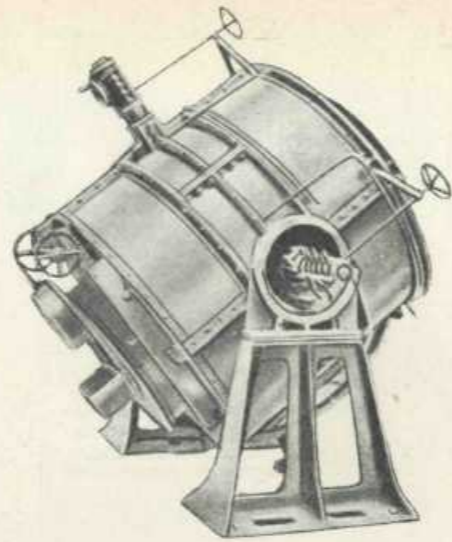
FIG. 10 - Forno Rennerfelt.
