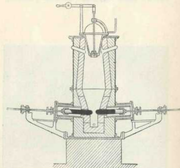
FIG. 6 - Forno Stassano. Tipo 1898.
