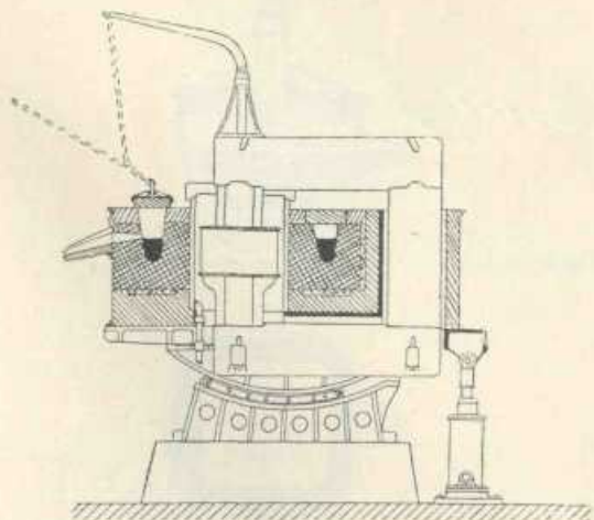
FIG. 3 - Forno ad induzione Kjelling.
