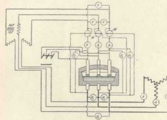
FIG. 14 - Forno Natusius (schema).
