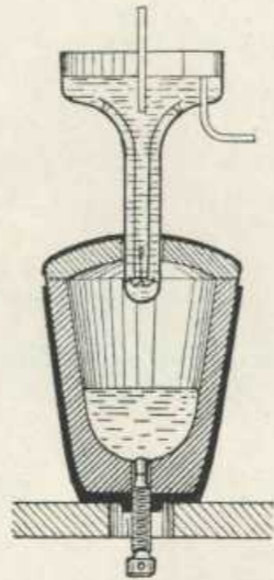
FIG. 11 - Crogiuolo Siemens ad arco diretto.
