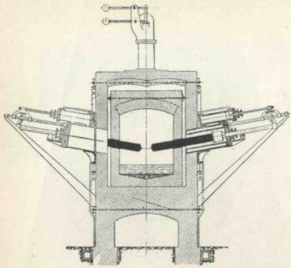
FIG. 7 - Forno Stassano. Tipo 1900.
