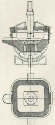
FIG. 12 - Forno ad arco diretto Girod.
