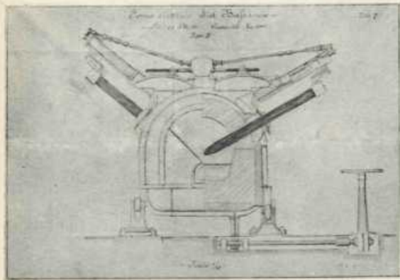
FIG. 8 - Forno Bassanese ( \frac{1}{2} vista, \frac{1}{2} sezione).
