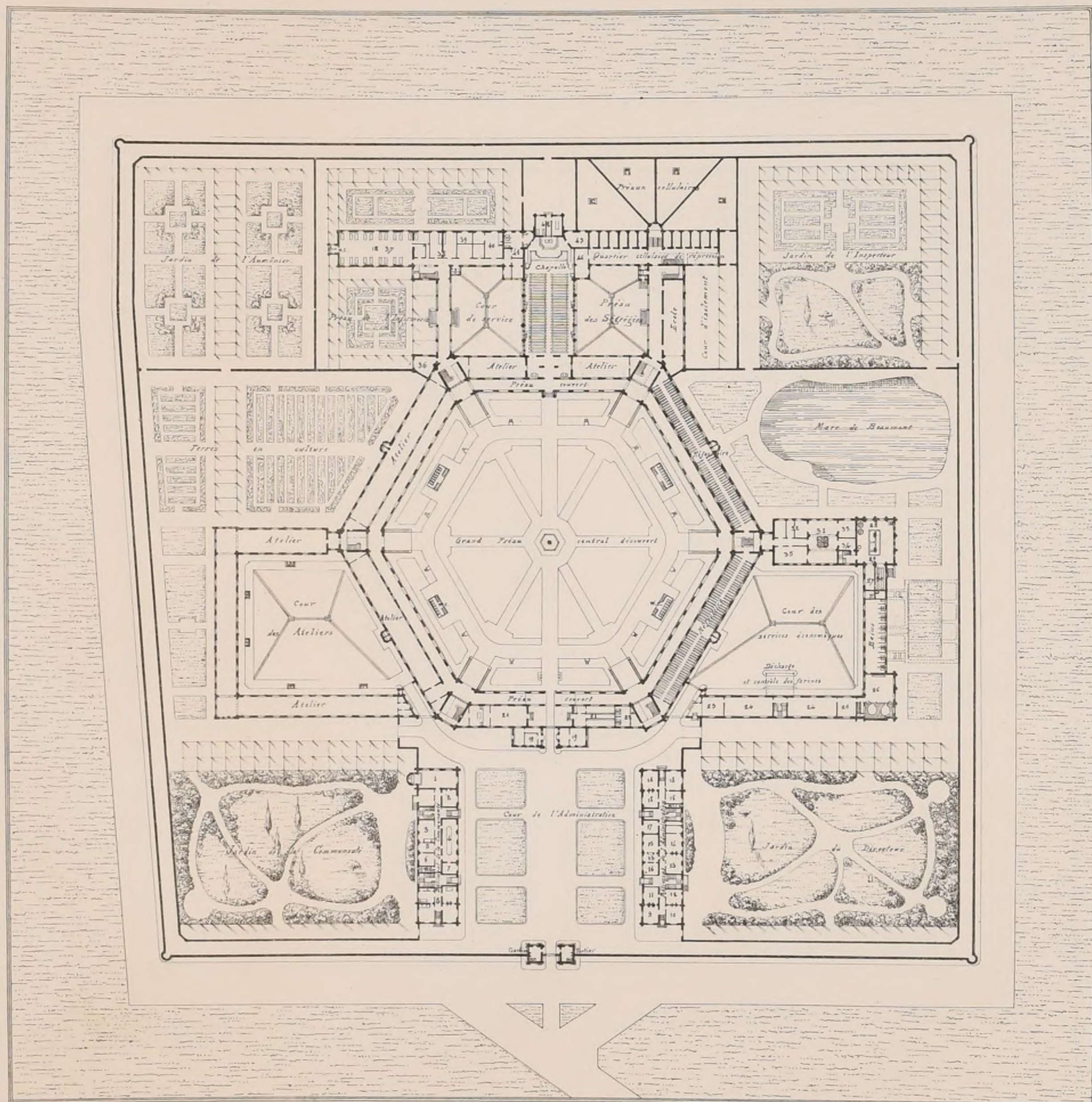
PLAN DU REZ-DE-CHAUSSÉE.
