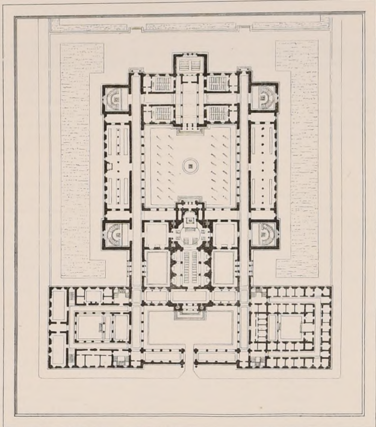
N° 10 M r ESQUIÉ élève de M r DAUMET
