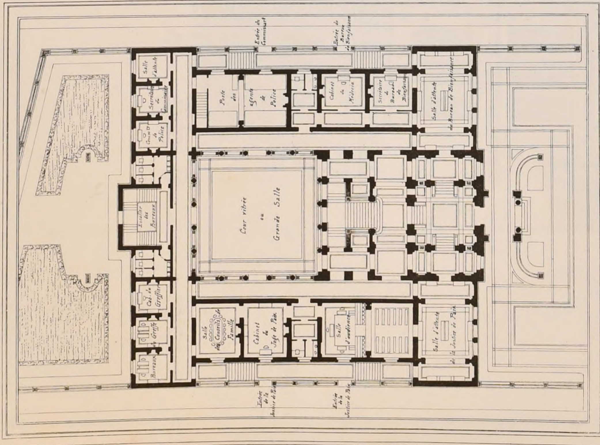
PLAN DU REZ-DE-CHAUSSEE
