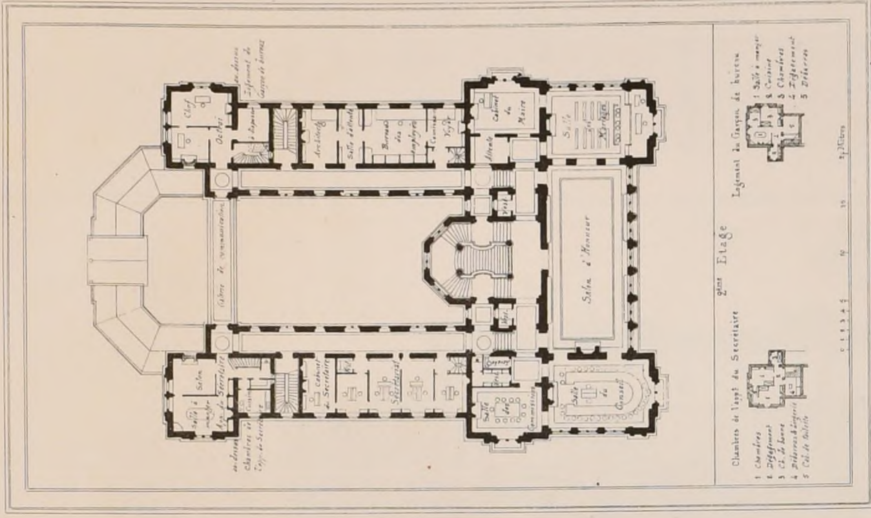
PLAN DU 1 er ÉTAGE
