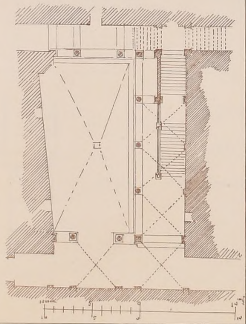
COUR DE L'ARCHEVÊCHÉ DE FLORENCE
