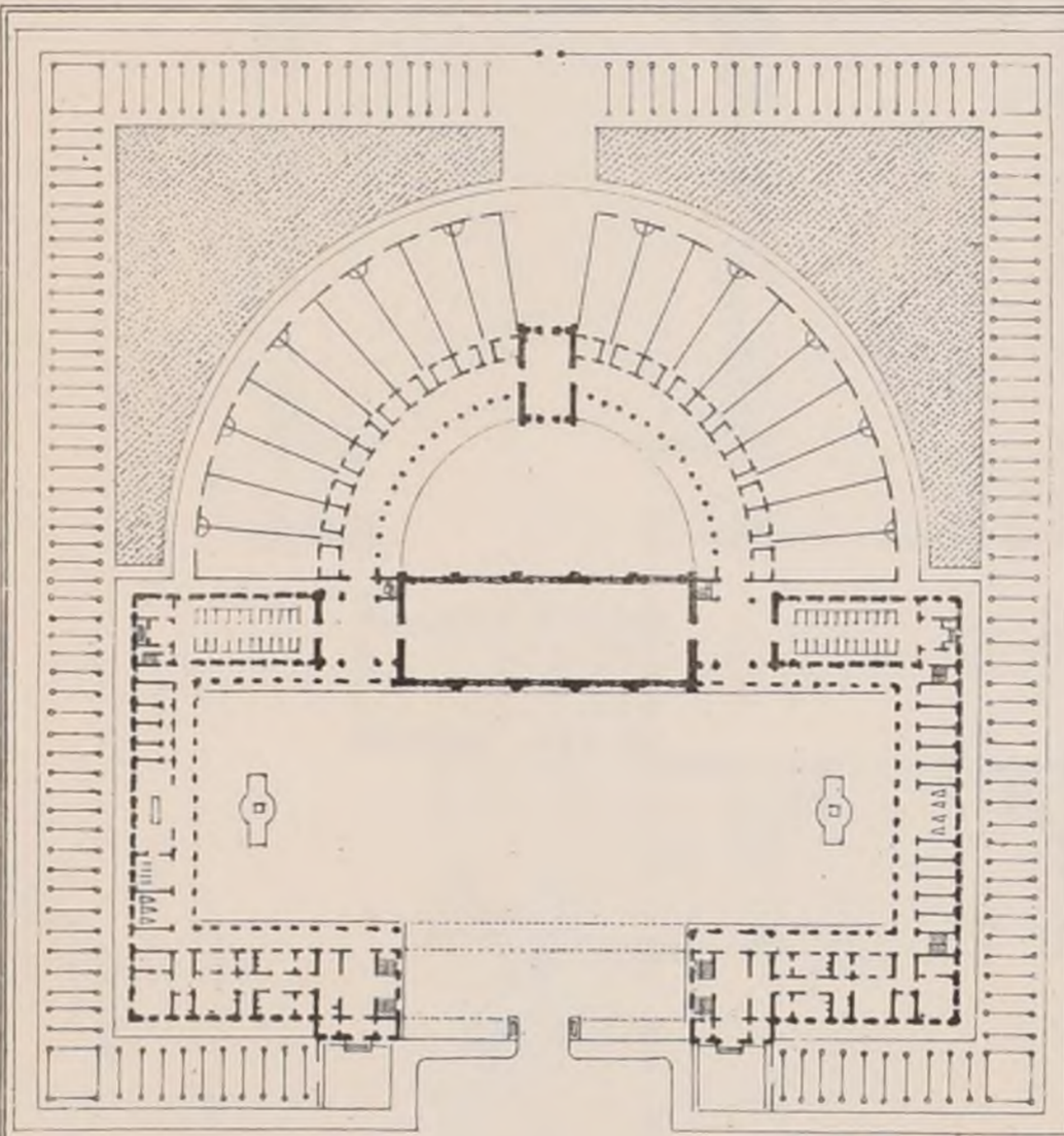
E D B-A Rendu de 1 re Classe. UN DÉPÔT DE CHEVAUX ÉTALONS. par M s DESLIGNIÈRES, élève de M rs Questel & Pascal. - 1 re Mention. Voir N° XII is F. 5.
