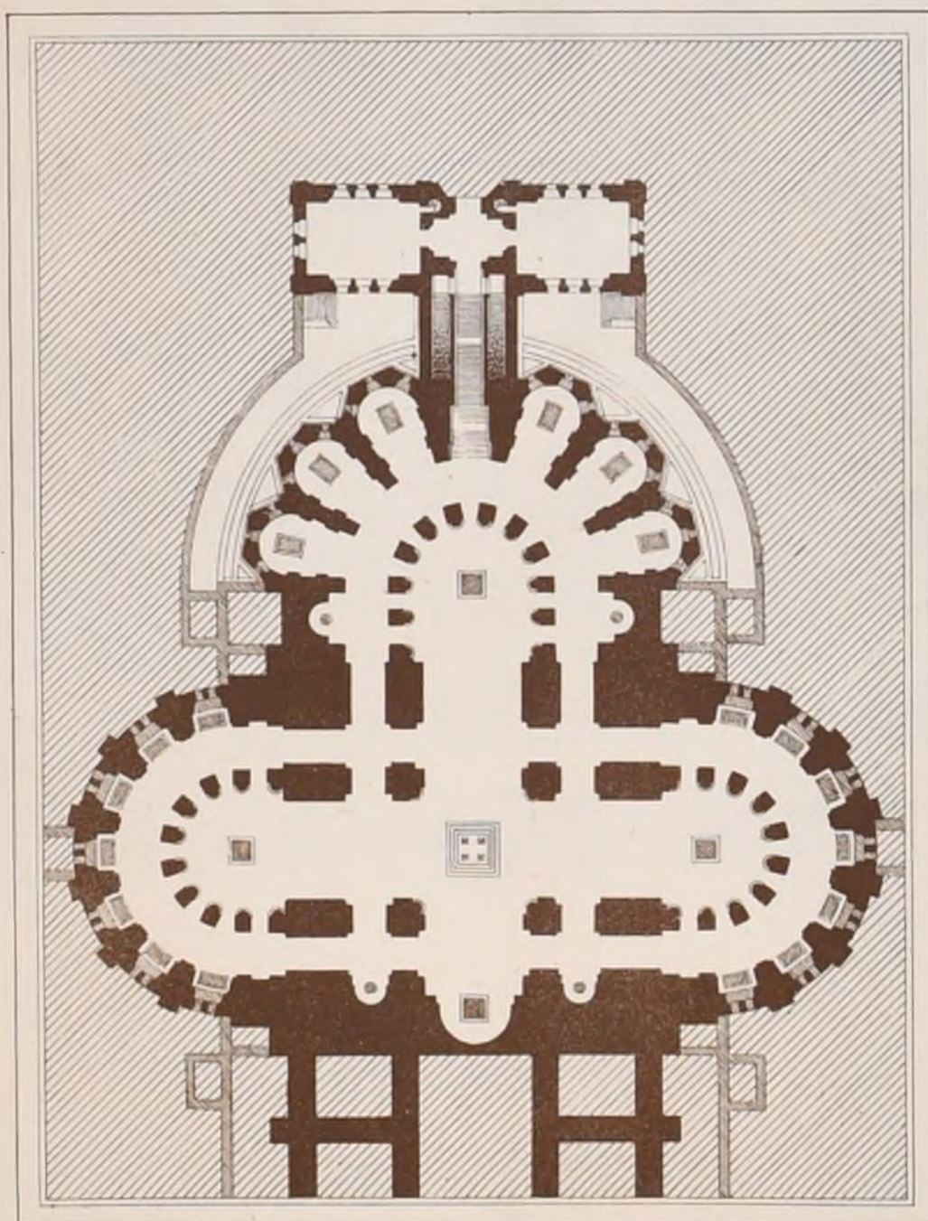
PLAN DE LA CRYPTE.
