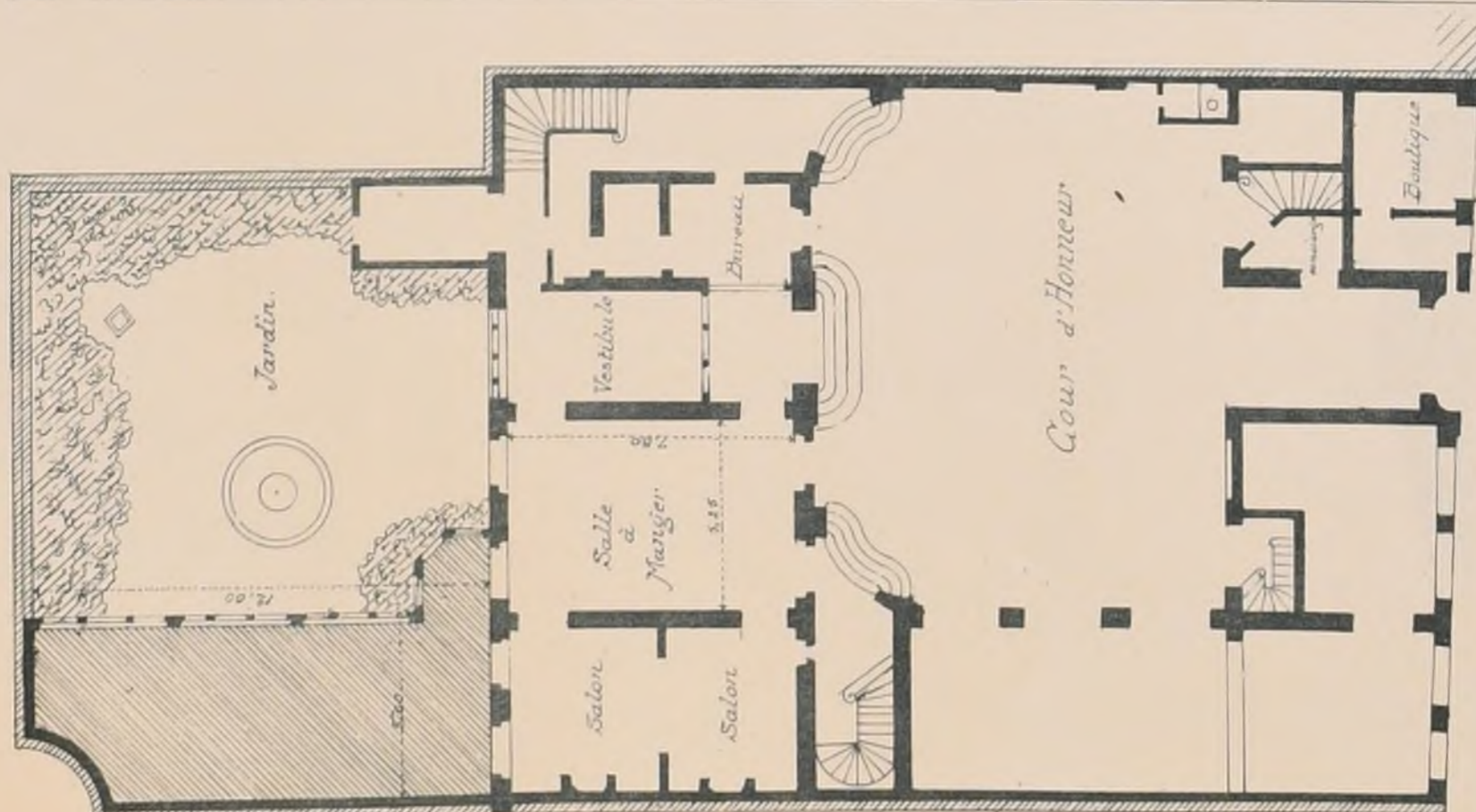
HÔTEL DES DUCS DE CHOISEUL, rue Coq-Héron. Exproprié en 1880 pour la reconstruction de l'Hôtel des Postes.
