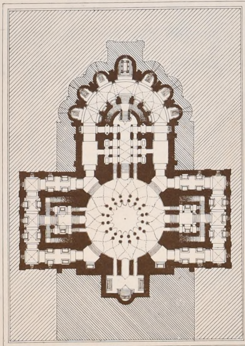
PLAN DE LA CRYPTÉ.
