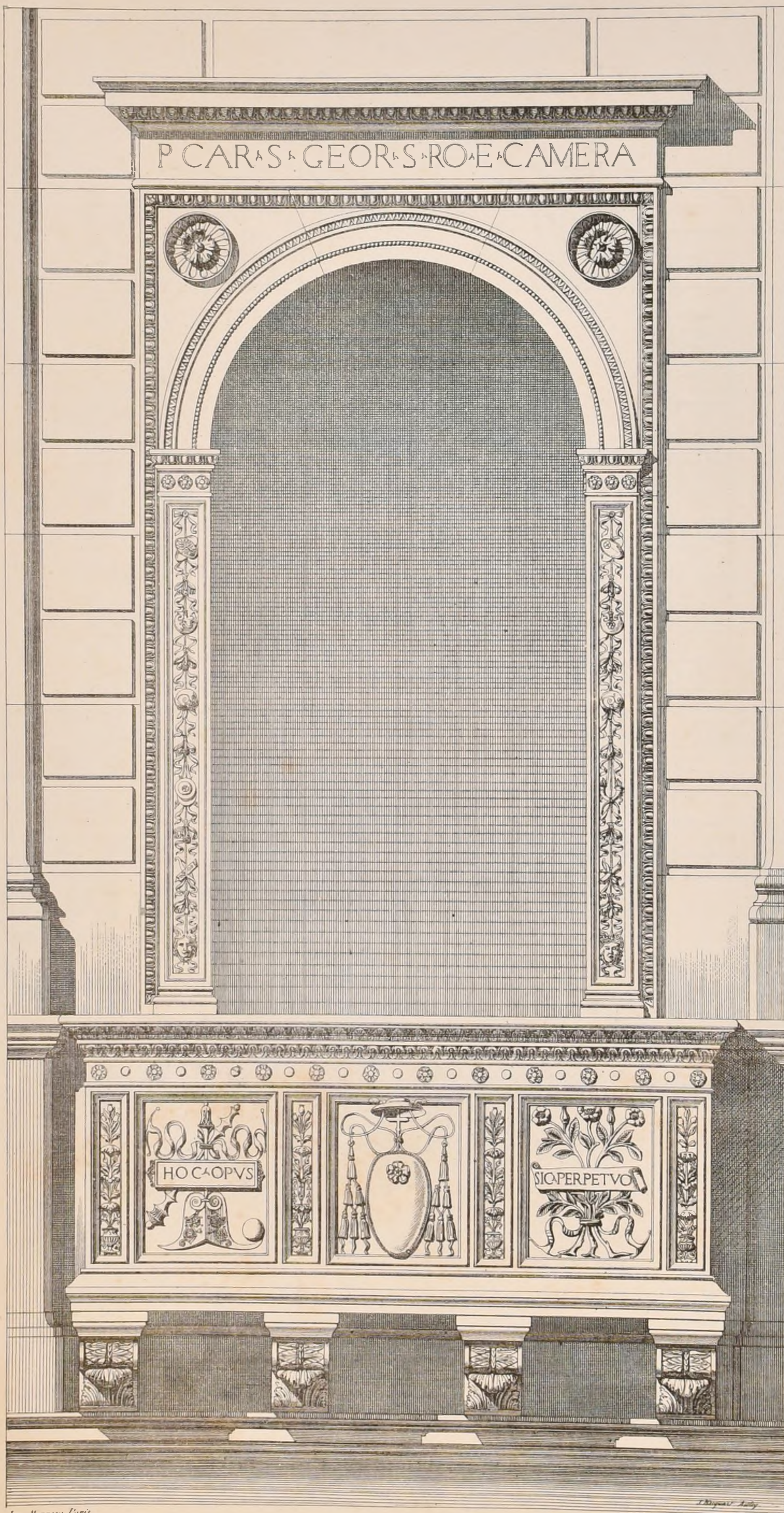
CROISÉE AU 1 er ETAGE DU PALAIS DE LA CHANCELLERIE A ROME relevée par M r ALBERT THOMAS
