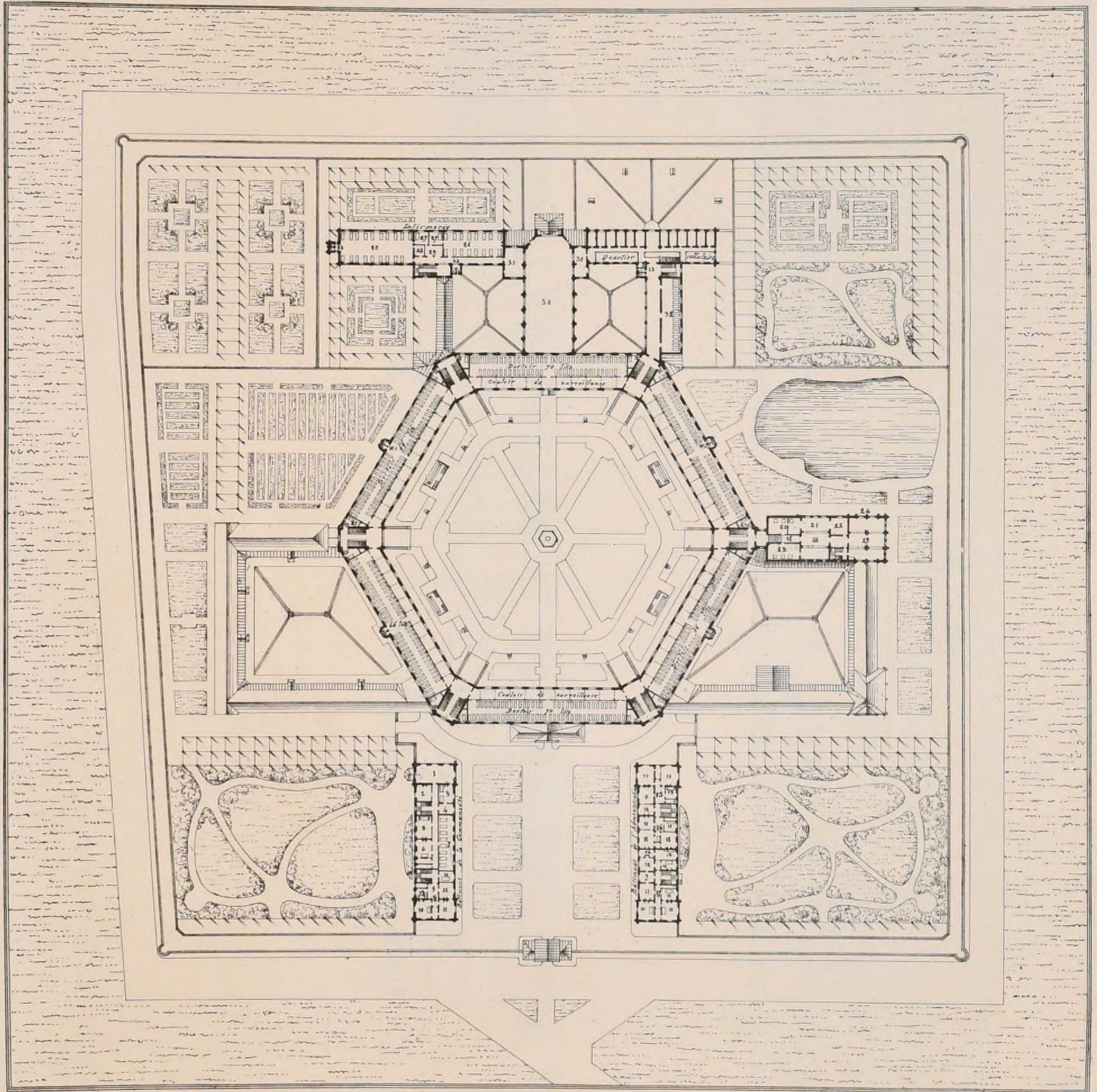
PLAN DU 1 er ÉTAGE
