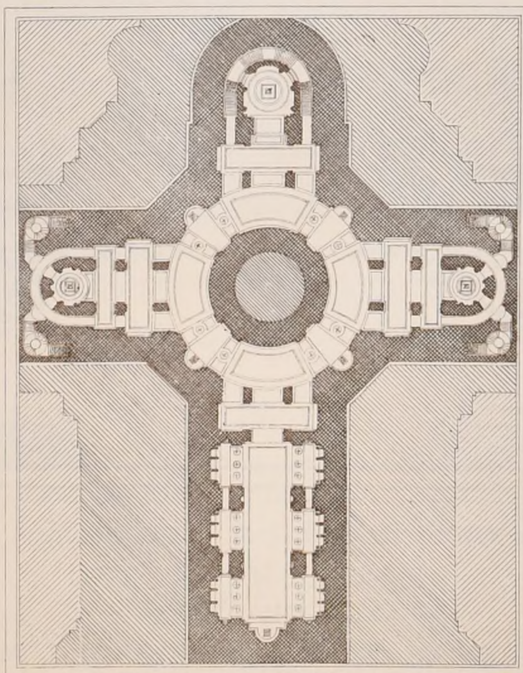
PLAN DE LA CRYPTÉ
