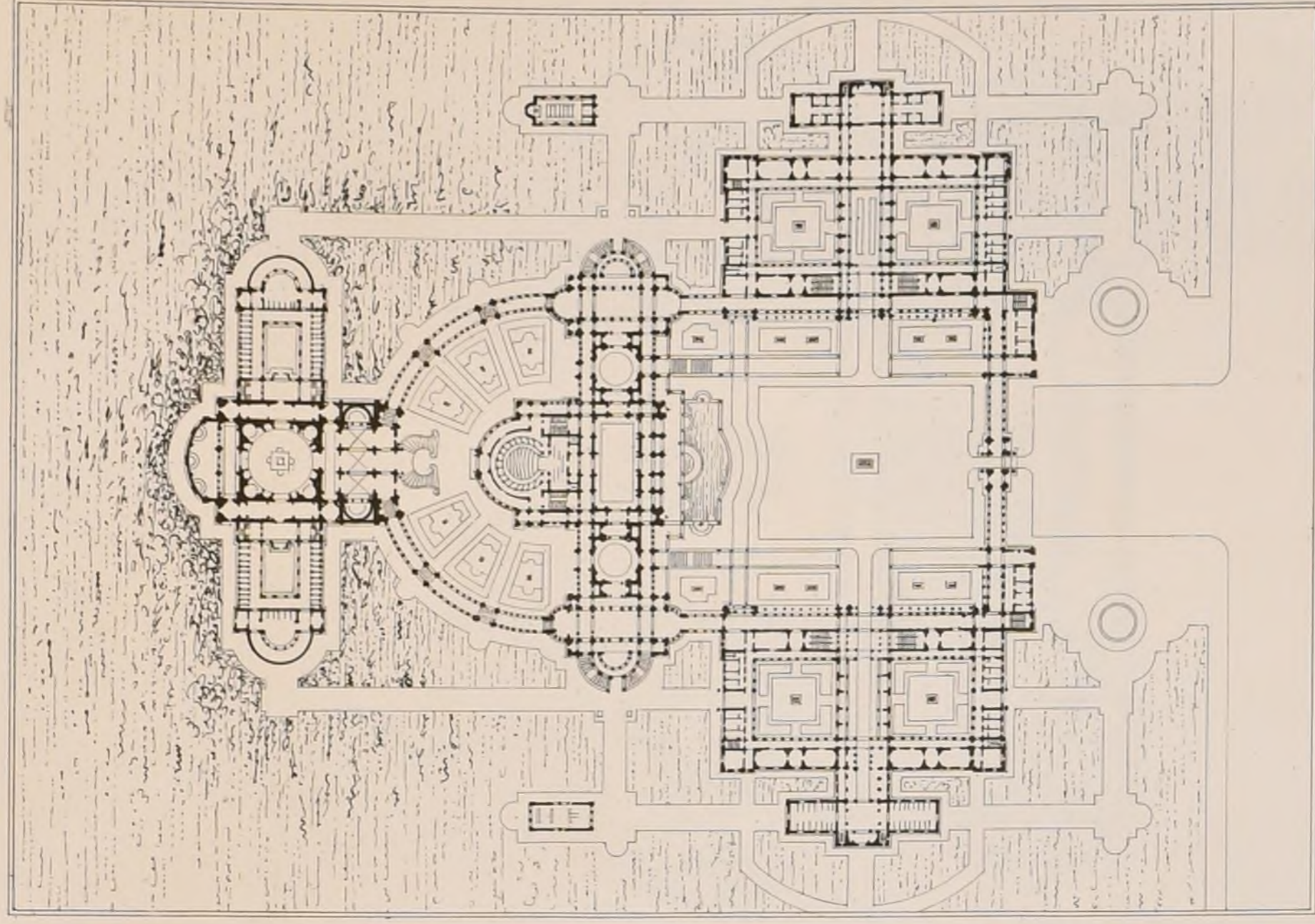
N o 3. M r HÉNARD, élève de M r HÉNARD.
