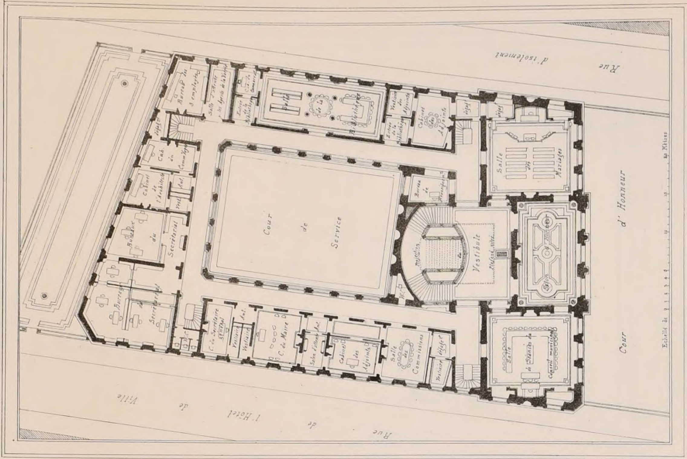
PLAN DU 1 er ÉTAGE
