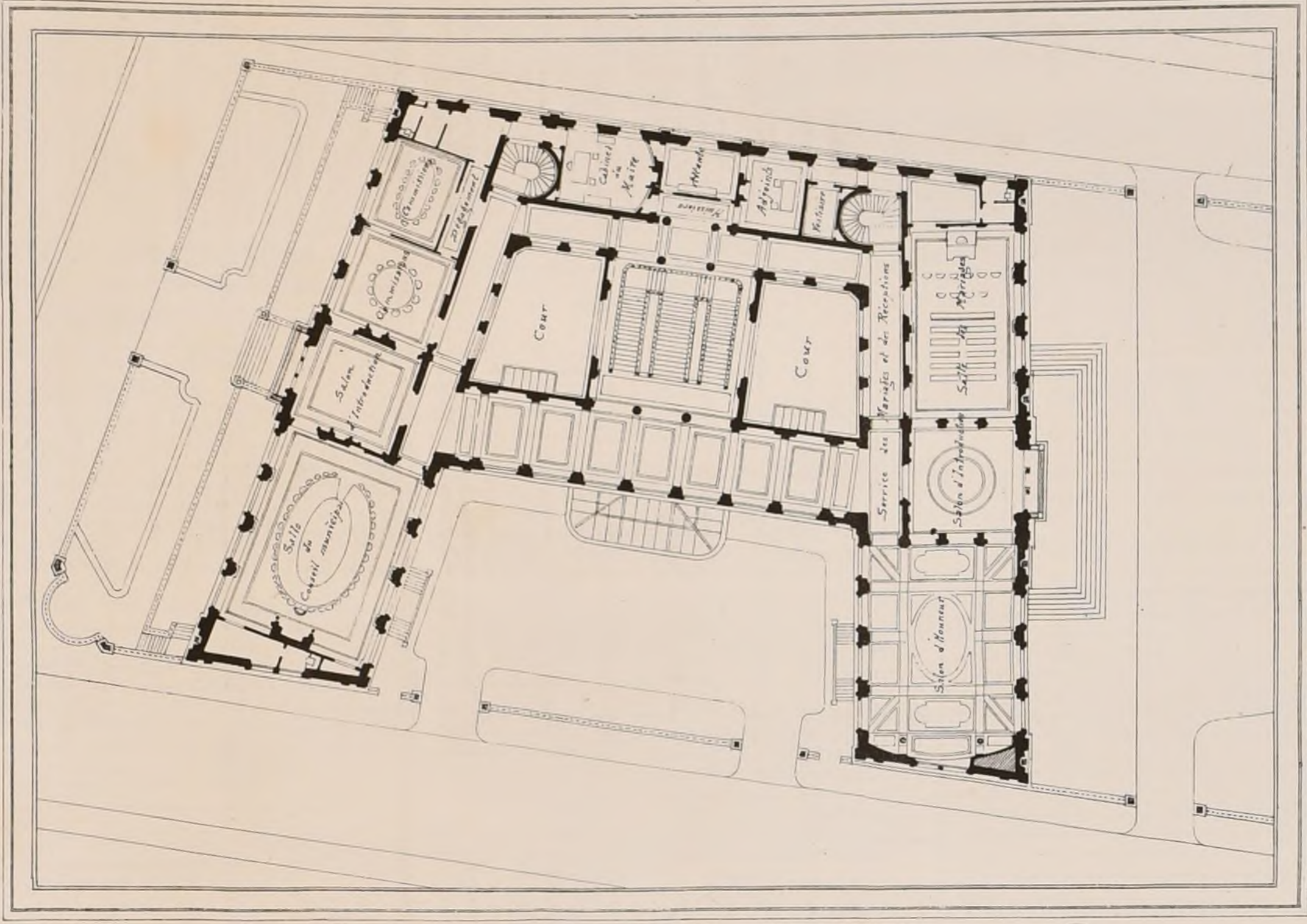
PLAN DU 1 er ÉTAGE
