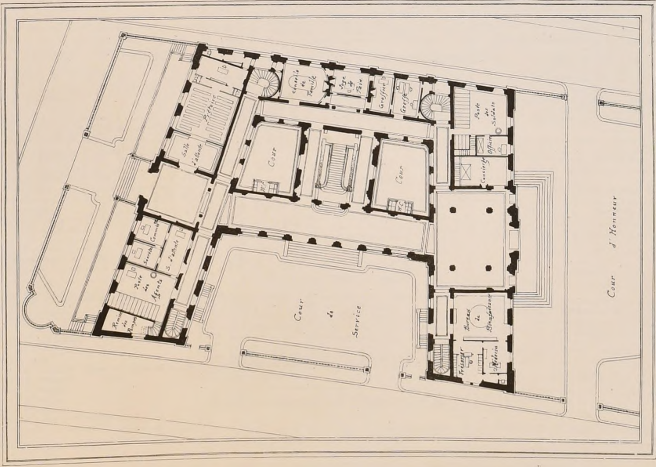
PLAN DU REZ-DE-CHAUSSÉE
