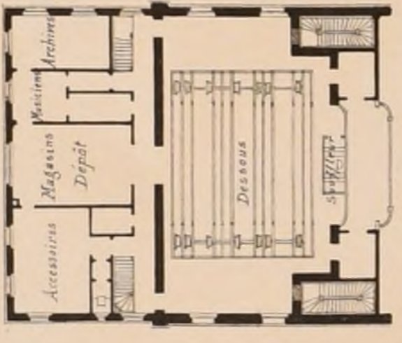
PLAN DE L'ENTRESOL
