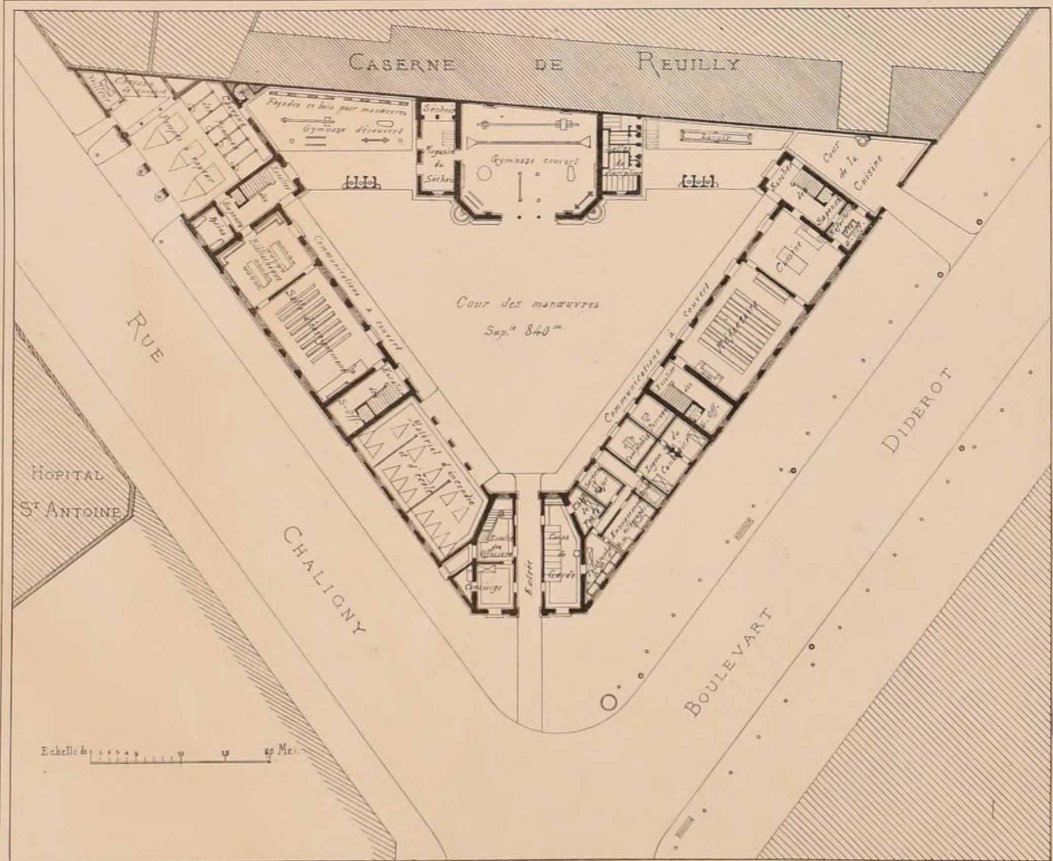
PLAN DU REZ-DE-CHAUSSÉE
