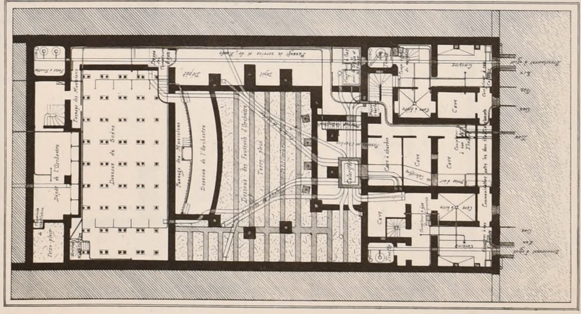
Sous-Sol
