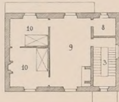
Plan du 1 er Etage.
