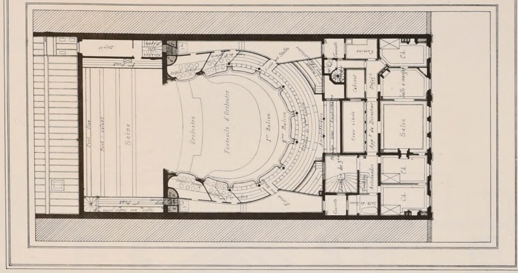
3 ème GALERIE
