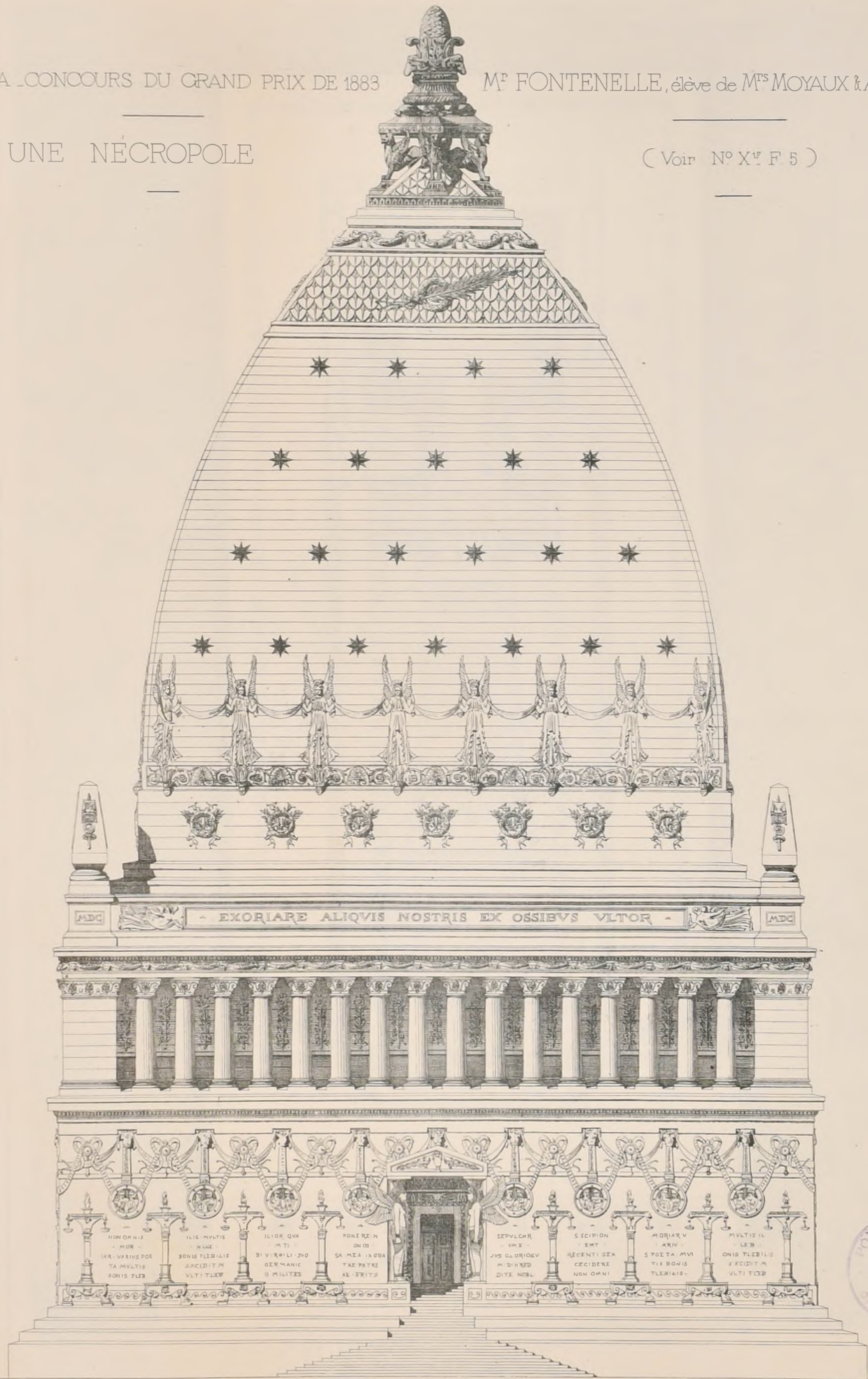
DETAIL DE L'ÉLEVATION DU MOTIF PRINCIPAL
