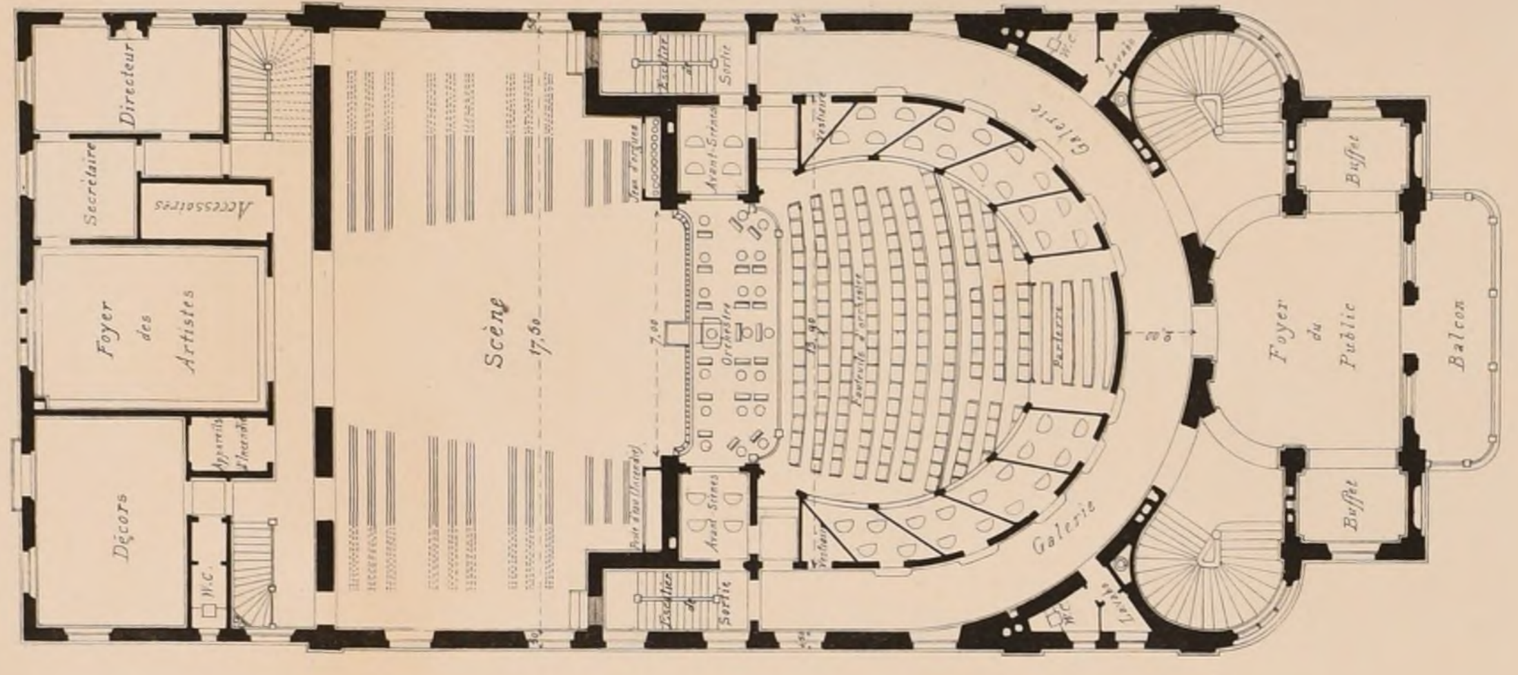
PLAN DU 1 er ETAGE
