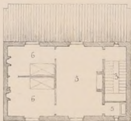
Plan du 1 er Etage.
