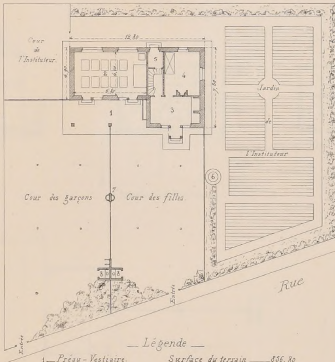
Plan.
