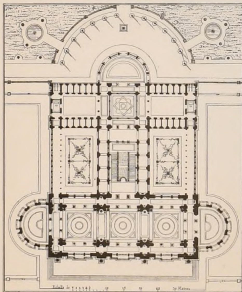
PLAN DU 1 ER ETAGE.
