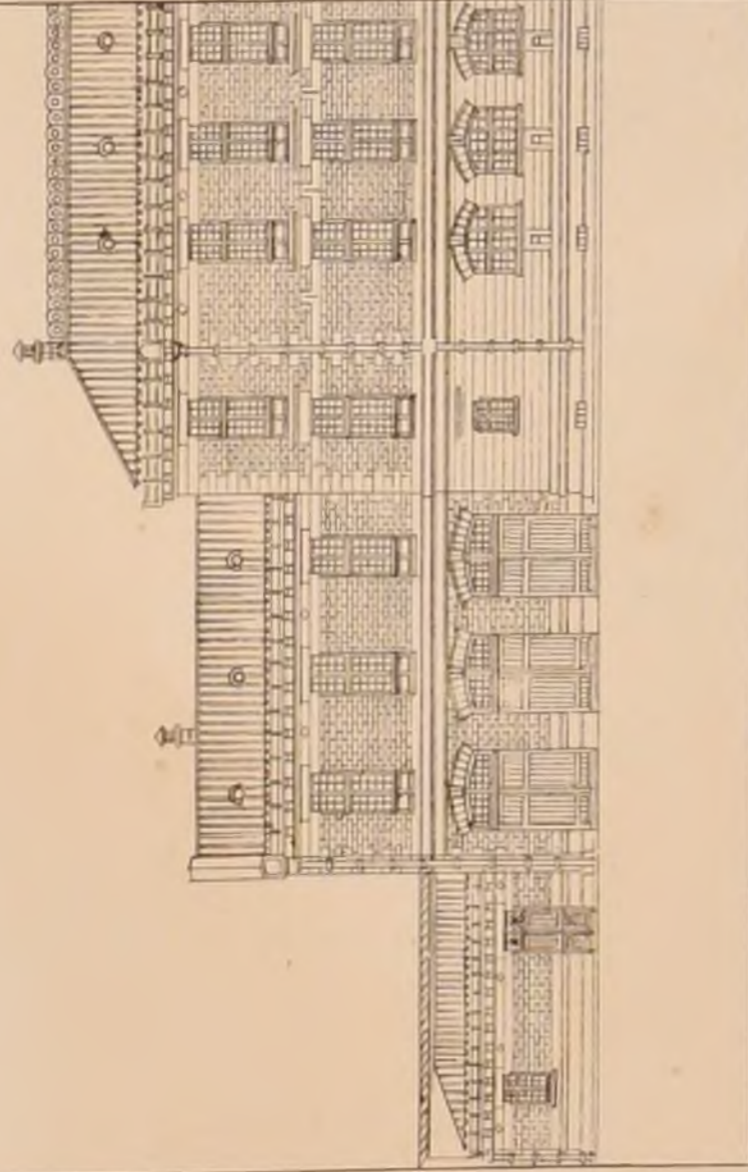
Partie d'ELEVATION sur la rue de Chaligny.
