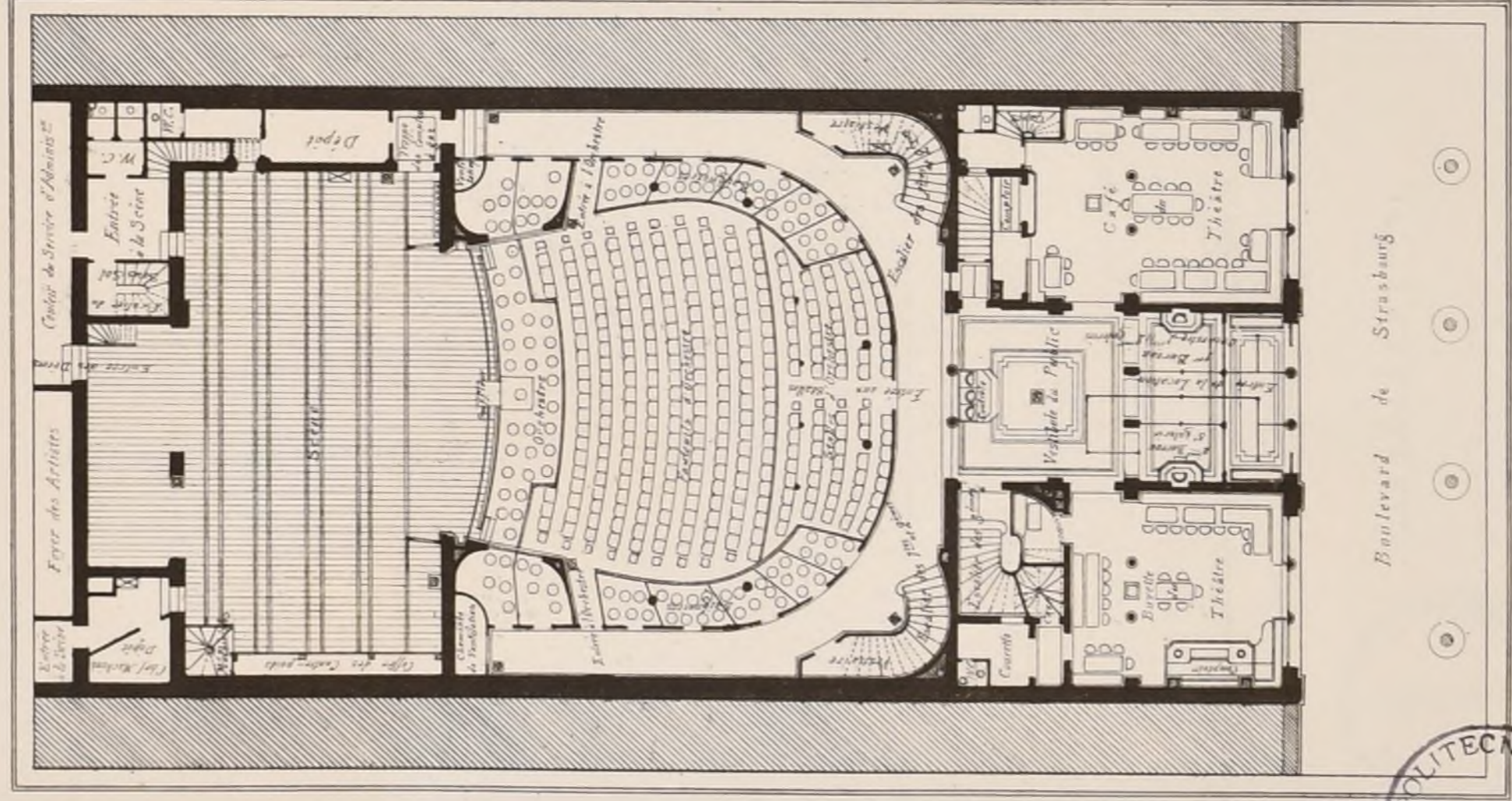
Rez-de-Chaussée
