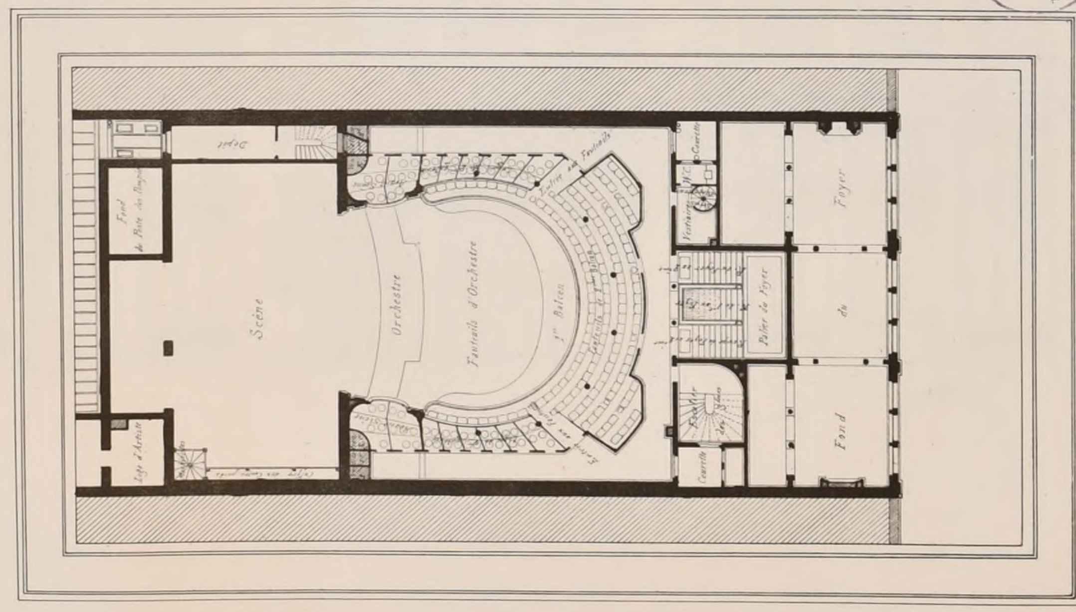
2 ème GALERIE
