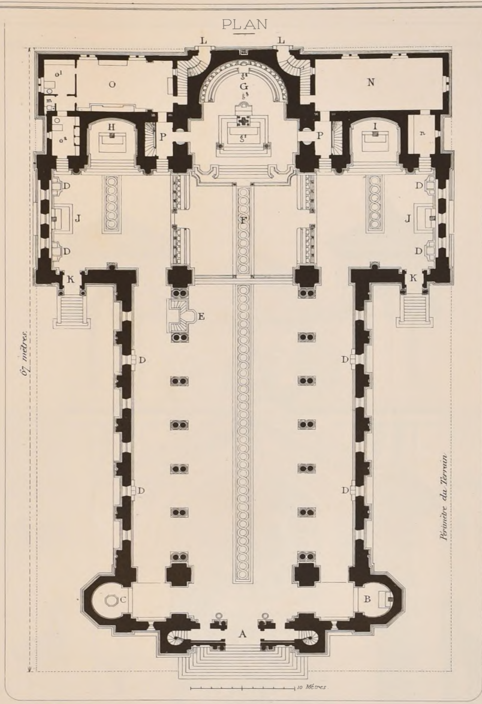
PLAN DES PARTIES HAUTES DE L'ÉGLISE
