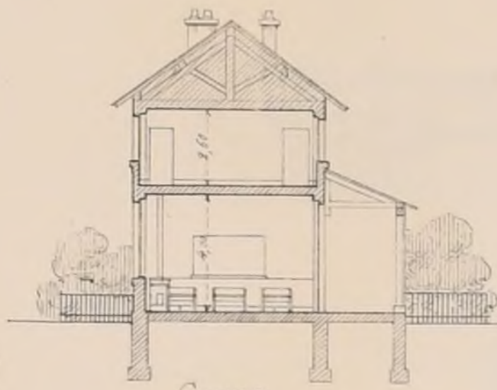
Coupe.
