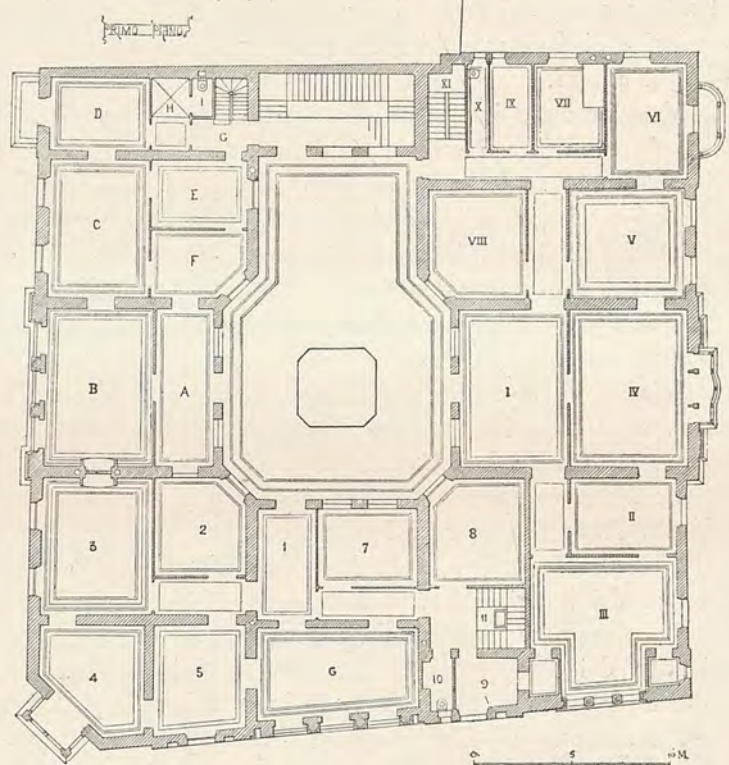
A. Vestibolo Ufficio Daira. — B. Salone per i Principi. — C. Studio per i Principi. — D. Camera di riposo. — E. Caposcrivano. — F. Salottino d'aspetto. — G. Entrata secondaria. — H. Toeletta. — I. Latrina. — 1. Vestibolo. — 2. Salottino. — 3. Salone. — 4, 5, 7, 8. Camere. — 6. Sala da pranzo. — 9. Bagno. — 10. Latrina. — 11. Scala di servizio e monta-piatti. — I. Vestibolo. — II. Salottino. — III. Salone. — IV. Sala da pranzo. — V, VI, VII, VIII. Camere. — IX. Bagno. — X. Latrina. — XI. Scala e monta-piatti per il servizio. Cucine, lavanderie, stanze servitù al piano delle terrazze.
