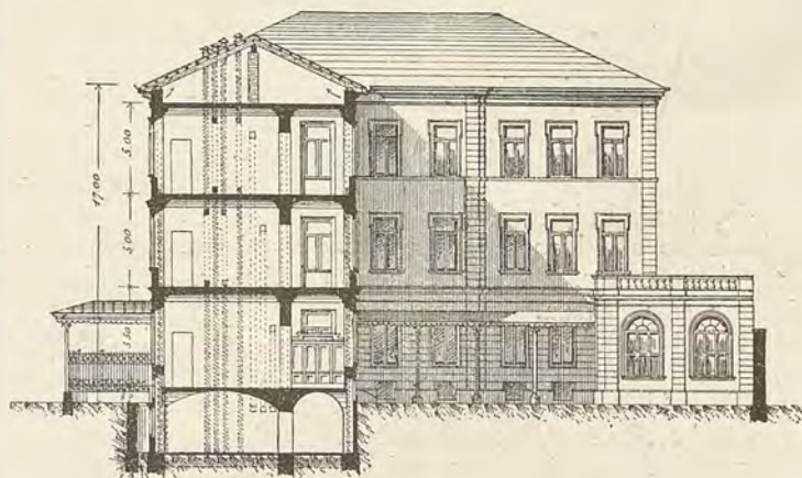
Serzione trasversale.
