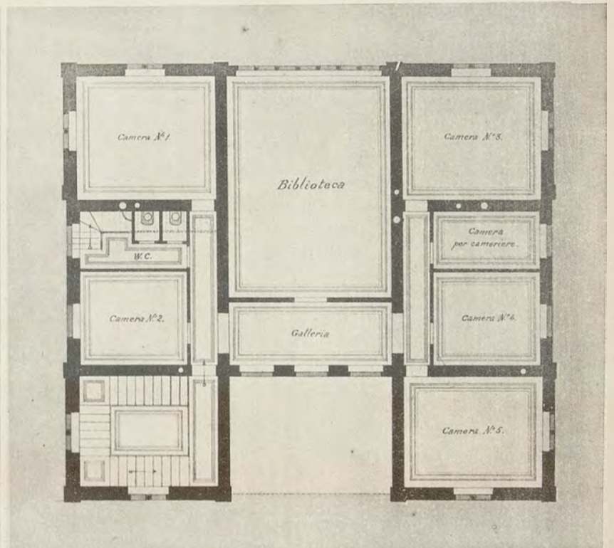
Secondo Piano Superiore (Scala 1:200)
