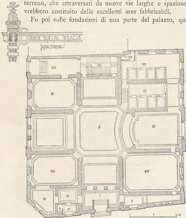
I. Vestibolo Club. — II. Guardaroba Signori. — III. Guardaroba Signore. — IV. Toeletta Signore. — V. Latrina. — VI. Salottino Signore. — VII. Salone di conversazione. — VIII. Sala da pranzo. — IX. Sala bigliardi. — X. Grande Salone. — XI. Palcoscenico. — XII e XIII. Camerino artisti. — XIV. Latrina. — XV e XVI. Vestibolo e scala per il Primo piano.
