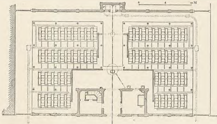
Pianta terrena.
