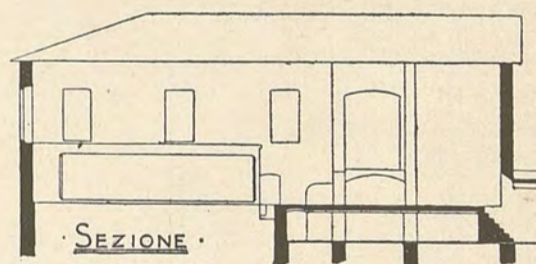
· LOCALE DELLE CALDAIE ·
