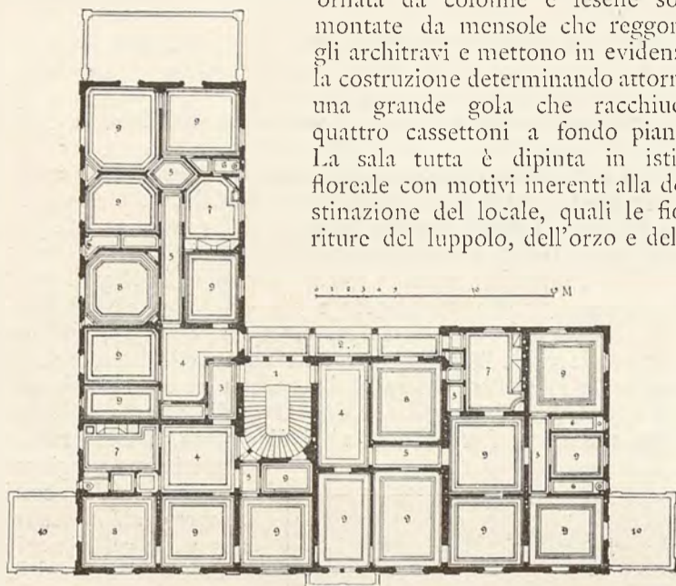
Pianta del secondo piano.
