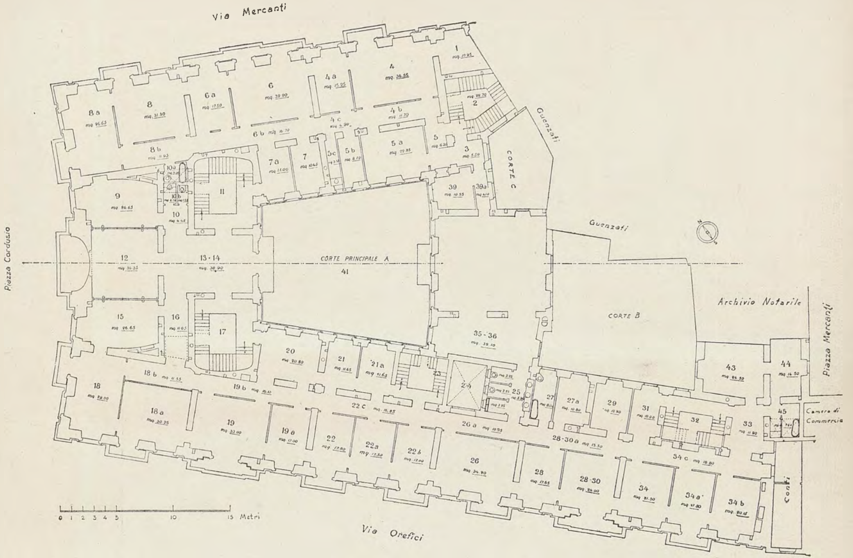
Pianta del I.º Piano.
