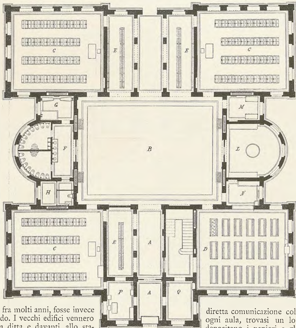
0 1 2 3 4 5 6 7 8 9 10 Metri
