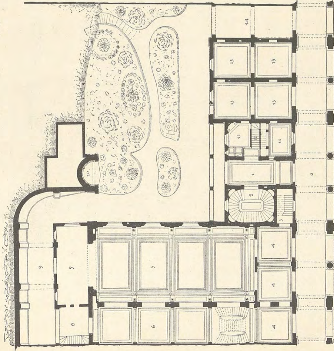
PIANO TERRENO.
