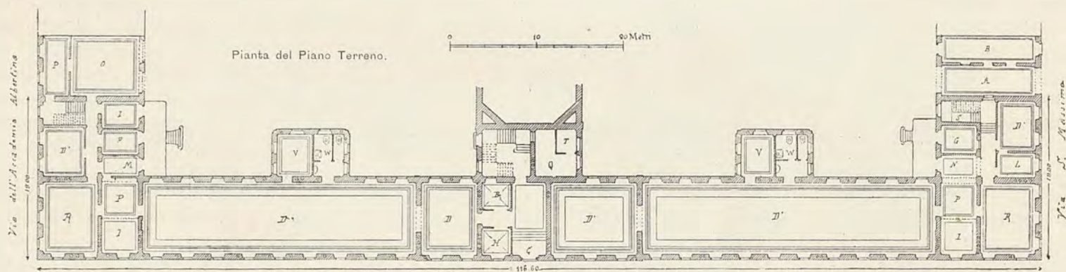
A. - Passaggio carraio. — B. B. - Portineria. — C. - Ingresso principale. — M. - Ingresso per incurabili (donne). — N. - Ingresso per incurabili (uomini). — P. P. - Passaggio. — I. I. - Gabinetto infermiere. — R. R. - Refettorio. — D. D. - Dormitòi incurabili (donne). — D' D' - Dormitòi incurabili (uomini). — S. S. - Scale di servizio. — F. F. - Servizio — G. - Camera di osservazione. — H. - Gabinetto suora. — L. L. - Camere di isolamento. — O. - Laboratorio. — P. - Laboratorio microscopia. — Q. - Laboratorio Radioscopico. — T. - Gabinetto fotografico. — W. W. - Cessi. — V. V. - Lavabos.
