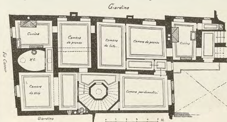
Pianta del Piano Sottterraneo
