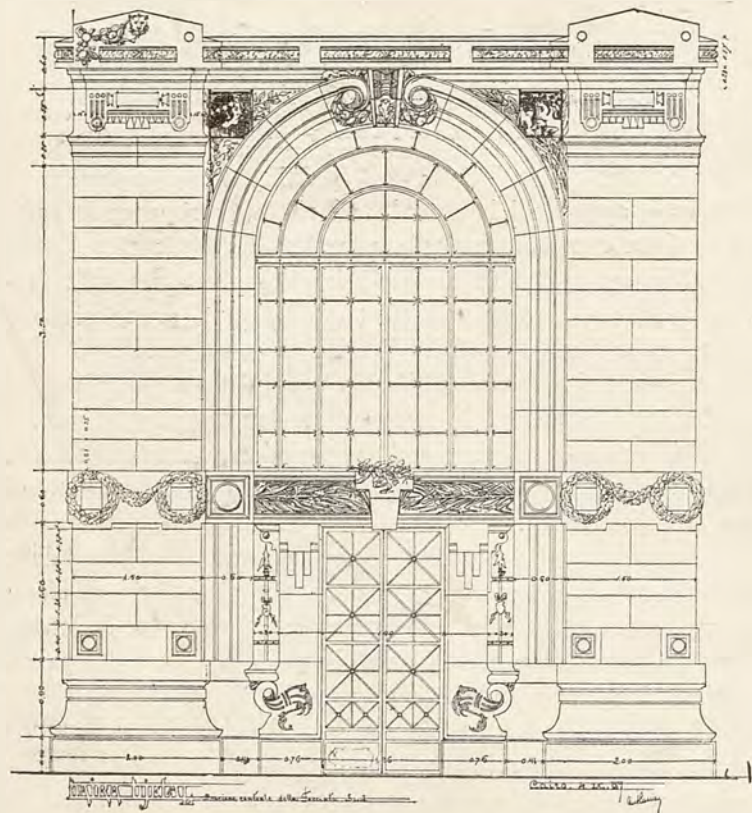
Porzione centrale della facciata sud.
