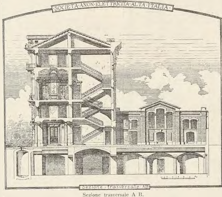
Sezione trasversale A B.
