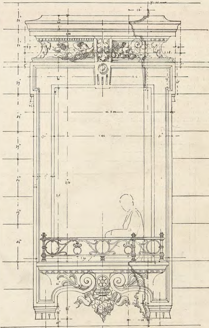
Finestra del secondo piano.
