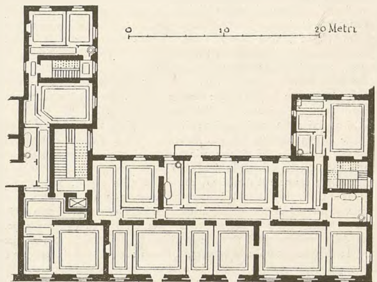
Pianta del Primo Piano Nobile.
