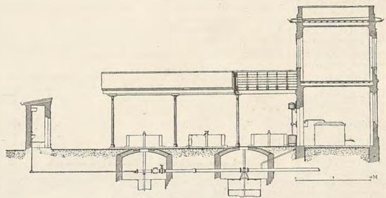
Sezione trasversale.
