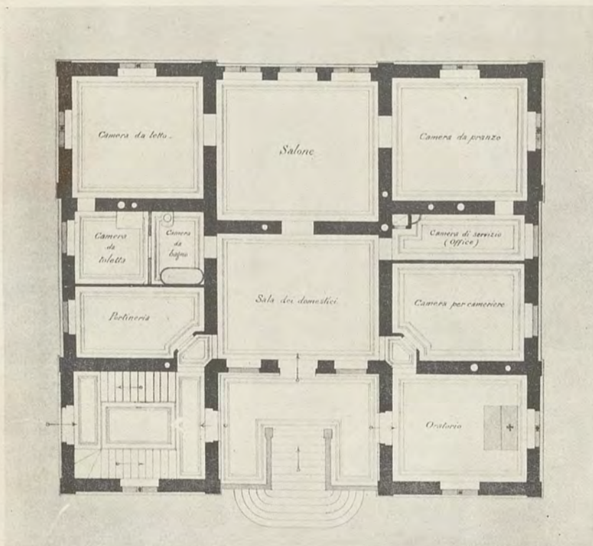
Piano Superiore (Scala 1:200)
