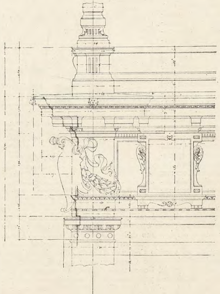
Motivo d'angolo del Cornicione ed attico.
