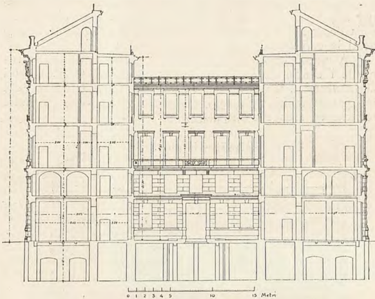
Schema della Sezione trasversale del Cortile principale.
