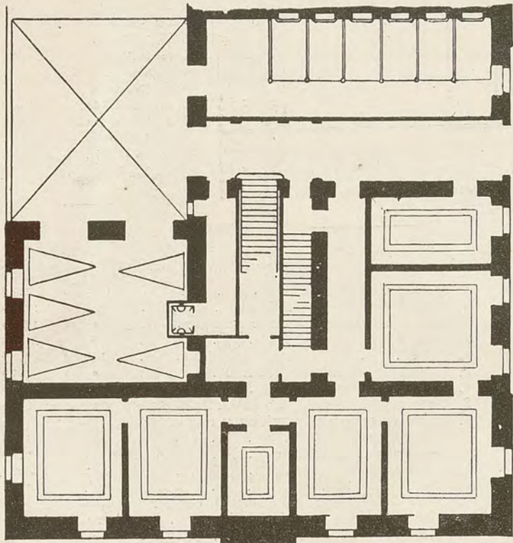
VIA S. BERNARDO Pianta del Piano Terreno
