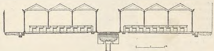
Sezione longitudinale.
