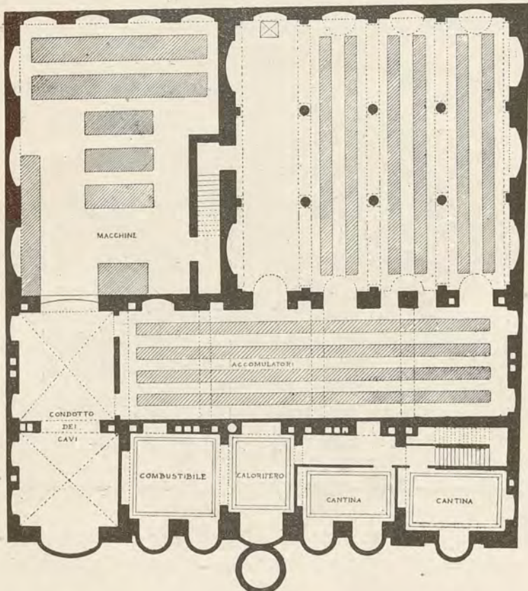
Pianta del Sotterraneo.
