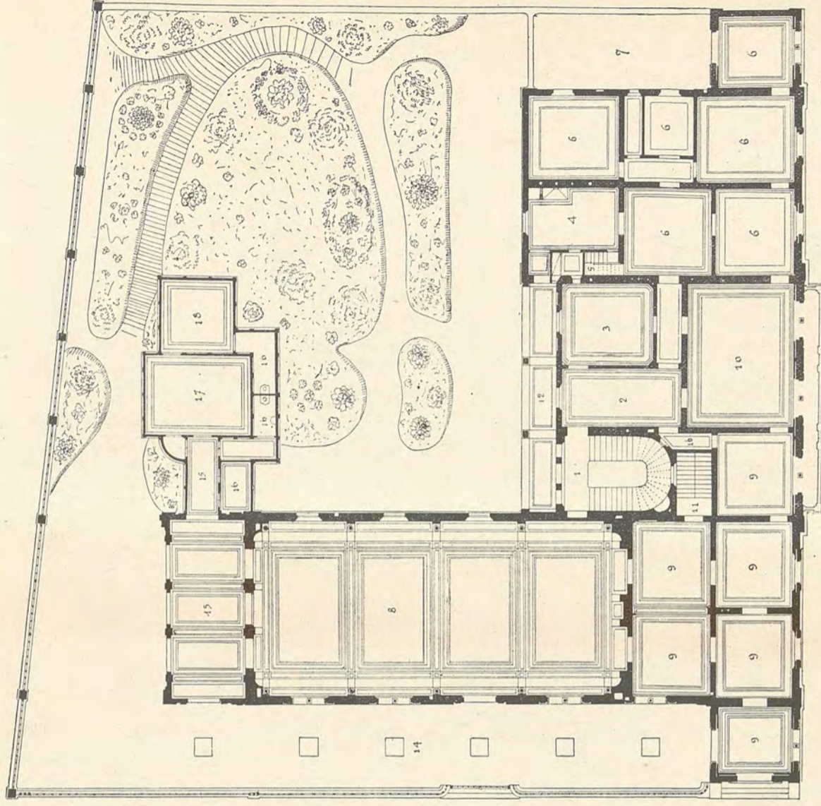
PRIMO PIANO.
