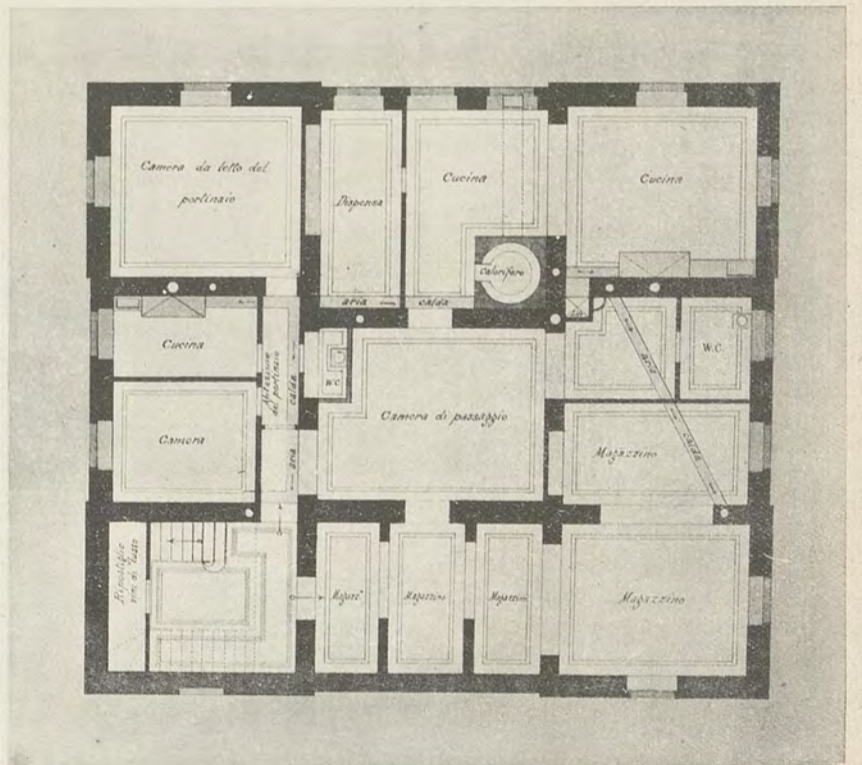
Piano Sotterraneo (Scala 1:200)
