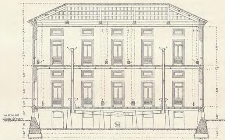
Sezione lungo l'asse di un' infermeria di medicina e di chirurgia.
